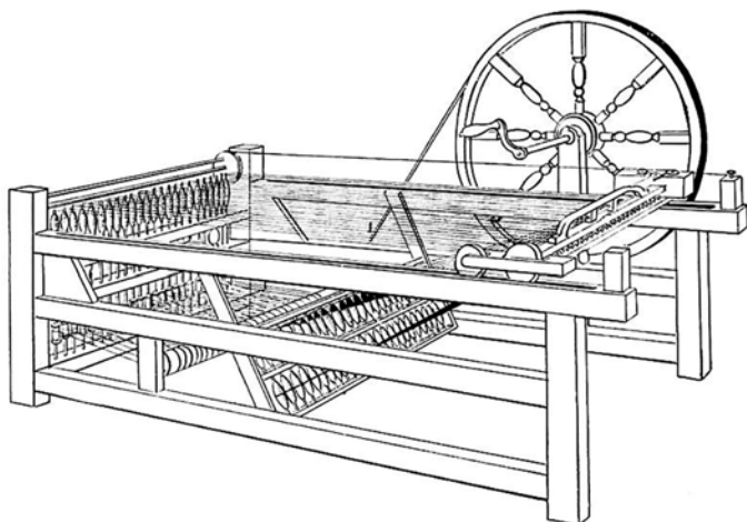
Die «Spinning Jenny» war die erste Spinnmaschine. Sie ersetzte anfänglich bis zu 20 Hand-Spinnerinnen. Die Jenny wurde mit einer Kurbel von Hand angetrieben, später kamen Wasserräder als Antrieb.
