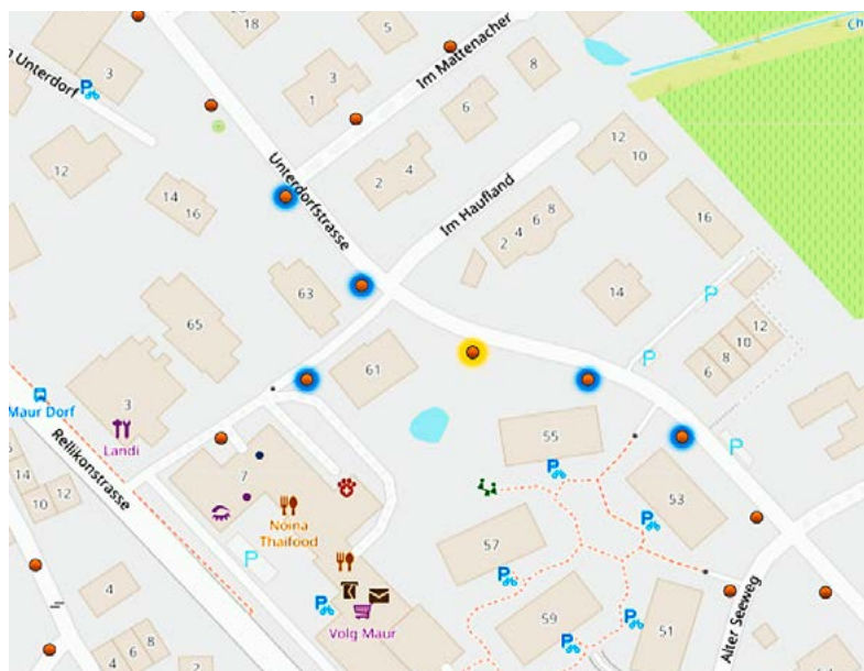
Die Grafik zeigt, wie die Leuchten miteinander kommunizieren: Die mittlere Leuchte erkennt ein Objekt und aktiviert die Leuchten auf beiden Seiten.
