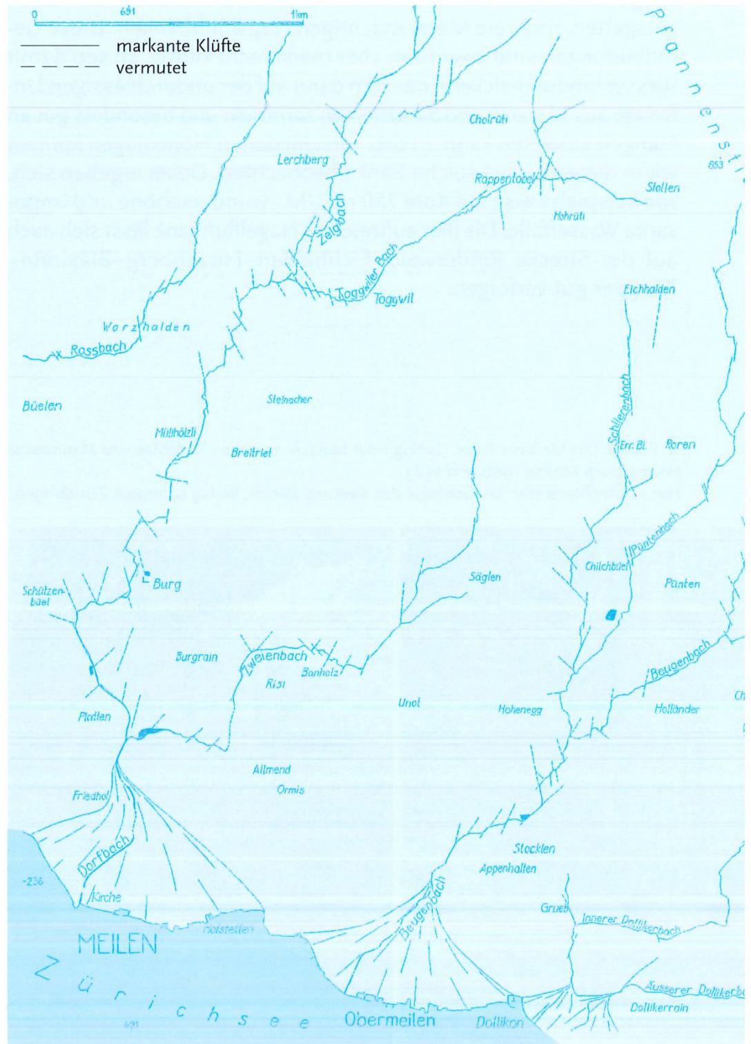
Abb. 1: Bedeutendere Klüfte mit Verstellung im Dorfbach- und im Beugentbachtobel, gezeichnet auf der Grundlage des Übersichtsplanes 2004, 1: 5000.
