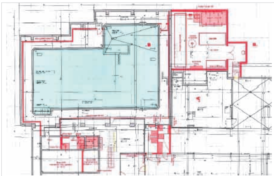
Lageplan mit projektierten Anlagen
