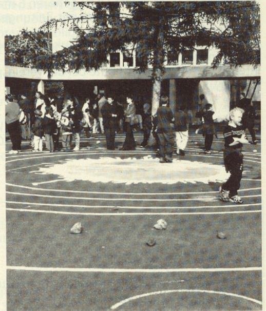
Das Sonnensystem
