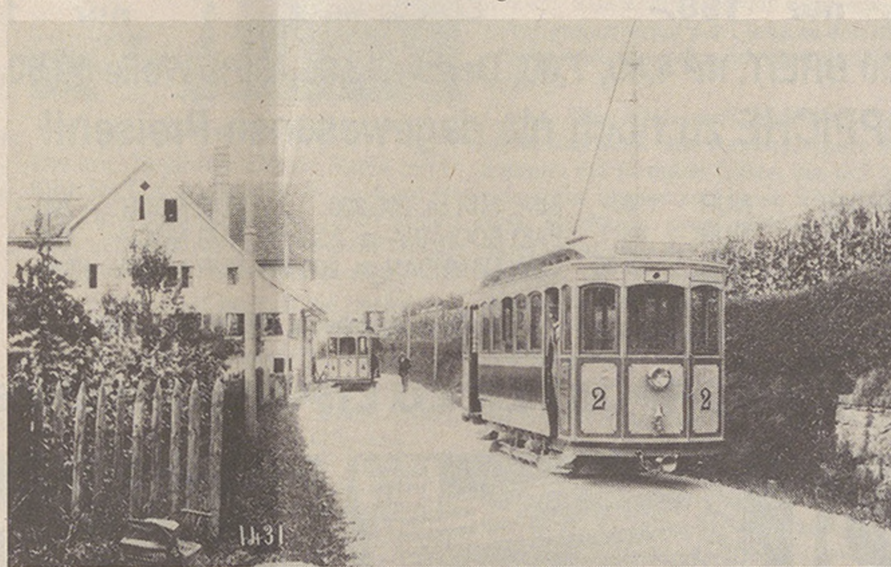
Der Motorwagen Ce 22 2 und 4 (SIG/MFO, 1898) der Strassenbahn Zürich-Höngg (Z-H) kreuzen sich bei der «Rotwand» im Eröffnungsjahr 1898. Foto: MFO, Archiv TMZ
