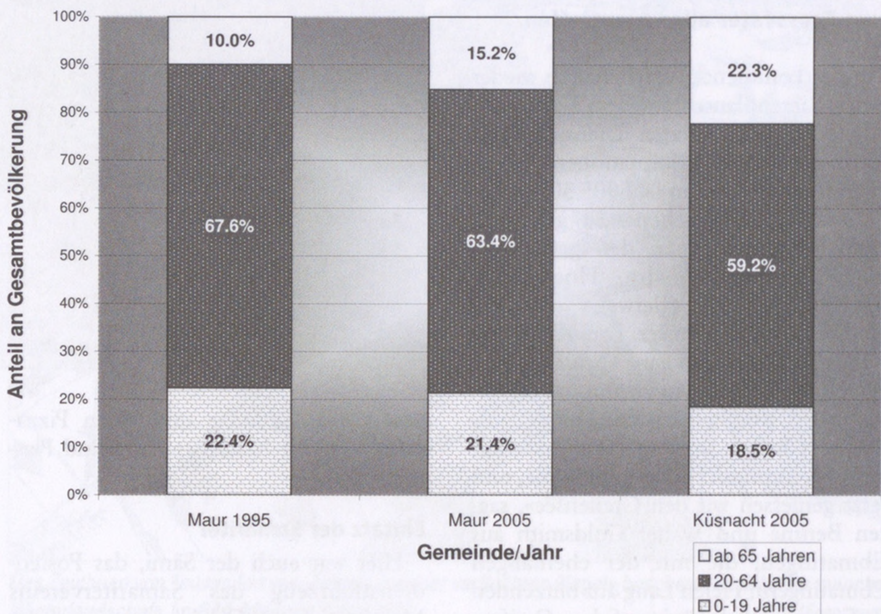
Altersstrukturvergleich
