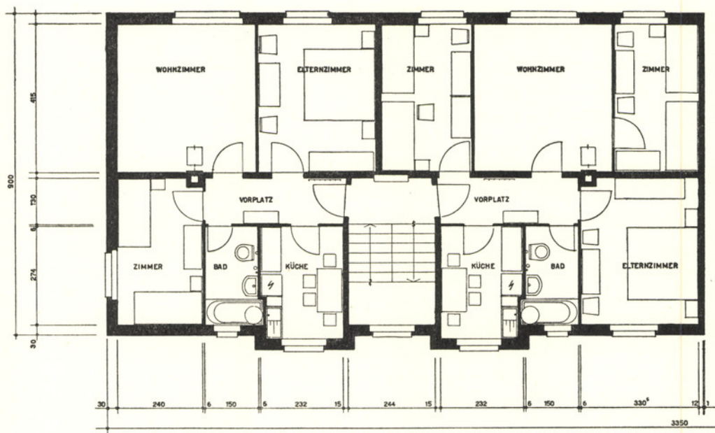
Grundriss der Wohnungen, wie sie an der Birchlenstrasse für Familien mit kleinem Einkommen im Baurecht erstellt werden sollen.
