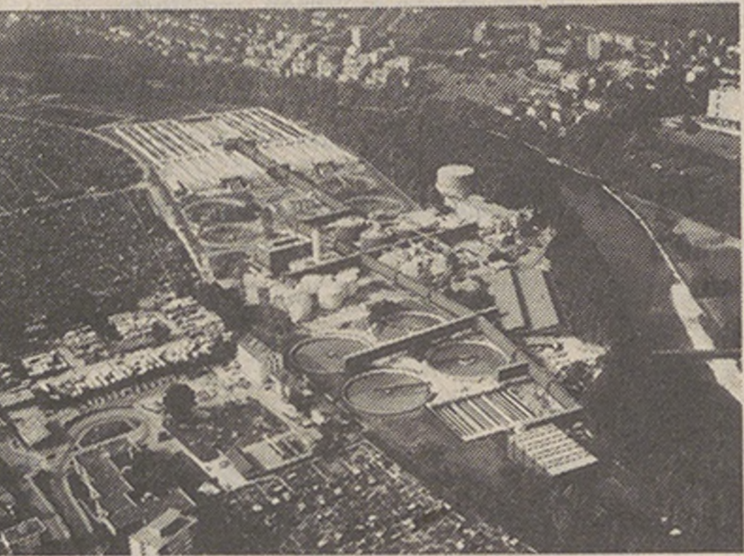
Erweiterte Kläranlage Werdhölzli: Im Vordergrund die mechanische Reinigungsstufe; in der Mitte die Tanks der Schlammbehandlung und das Betriebsgebäude mit dem Kamin der Energiezentrale. Im Hintergrund die biologische Reinigungsstufe mit der eingebetteten Filtrationsstufe (ganz oben im Bild).
