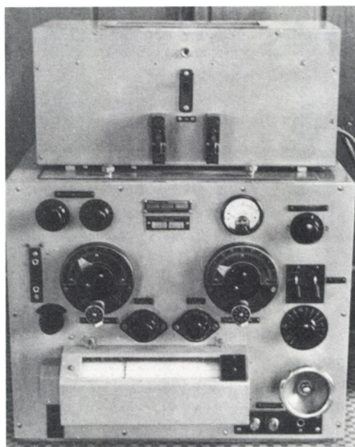
Der Marconi-Kurzwellenempfänger Typ RG34 von 1933 zeigte schon ein moderner anmutendes Design.
