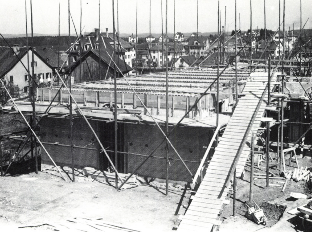
Neues Primarschulhaus Dorf B im Bau.
