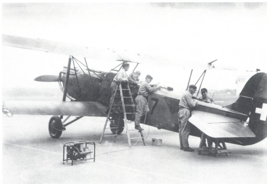
Abstimmen des Flugfunkgerätes FG-IV am Flugzeug Fokker CV, im Einsatz ab 1933 als Zweisitzer für Aufklärung und Erdkampf. Fk Mech Rekrut Kurt Bolliger arbeitet am Antennenabstimmgerät (Zweiter von rechts).
