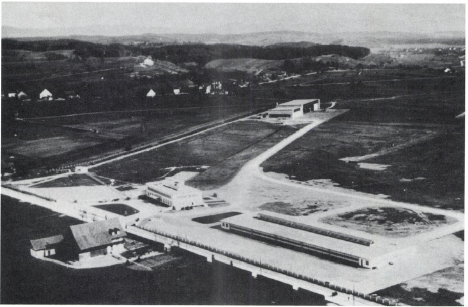
Die eben fertiggestellten Anlagen und Gebäude des Zivilflugplatzes Dübendorf-Zürich 1932.
