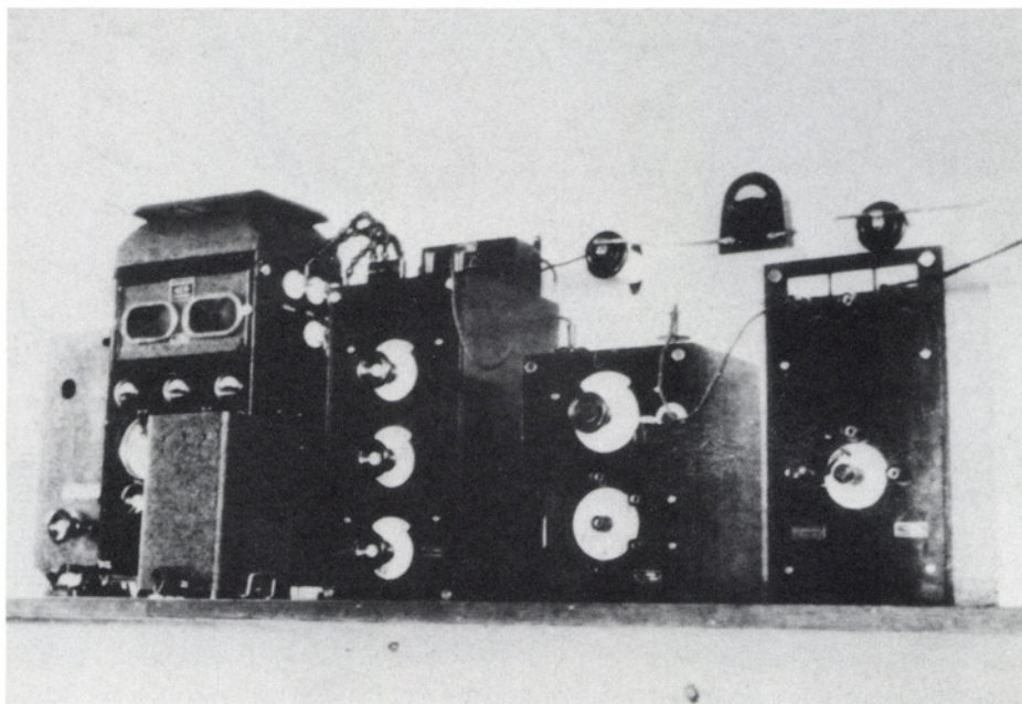
Die erste einfache Apparatur in Kloten hatte eine Sendeleistung von einem Kilowatt.
