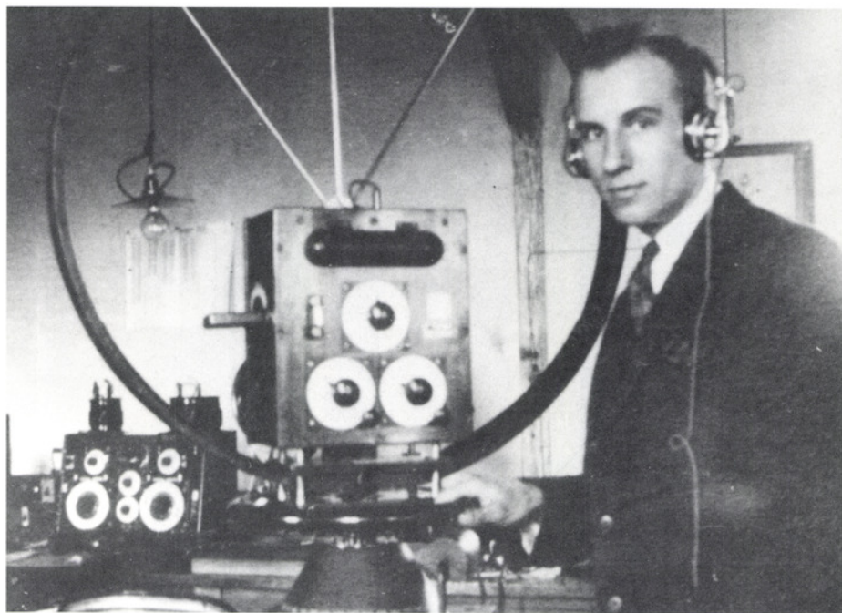
1925 erhielt Dübendorf erstmals eine Peilausrüstung in Form eines tragbaren Telefunken-Radiopeilers Typ E 276. Er war 1,2 m hoch und um 360 Grad drehbar.
