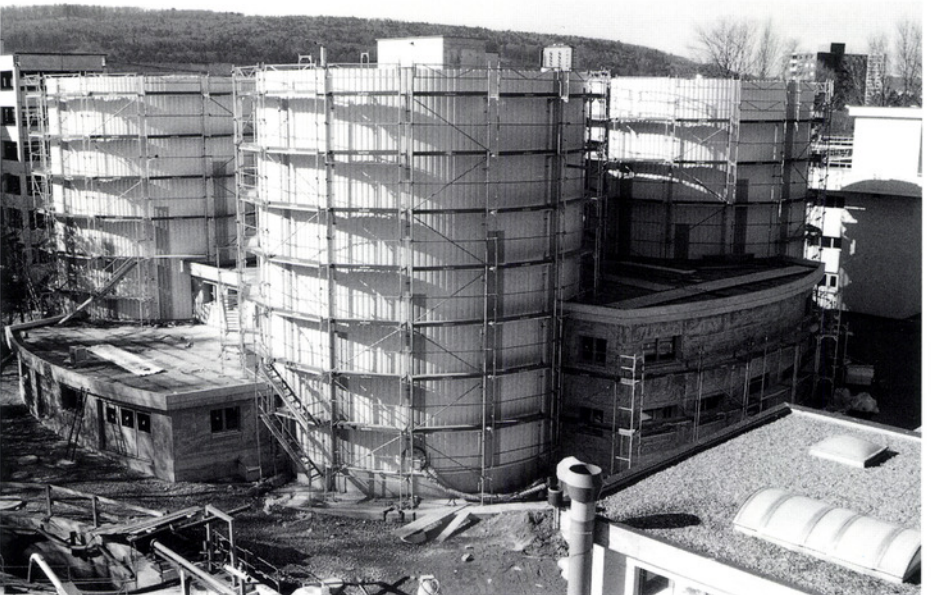
Bau der vier zur Schlammfäulung und Klärgasgewinnung dienenden Faultürme, die für ein Schlammvolumen von je 1400 Kubikmetern ausgelegt sind. In den Zwischenräumen ist das Betriebsgebäude entstanden.
