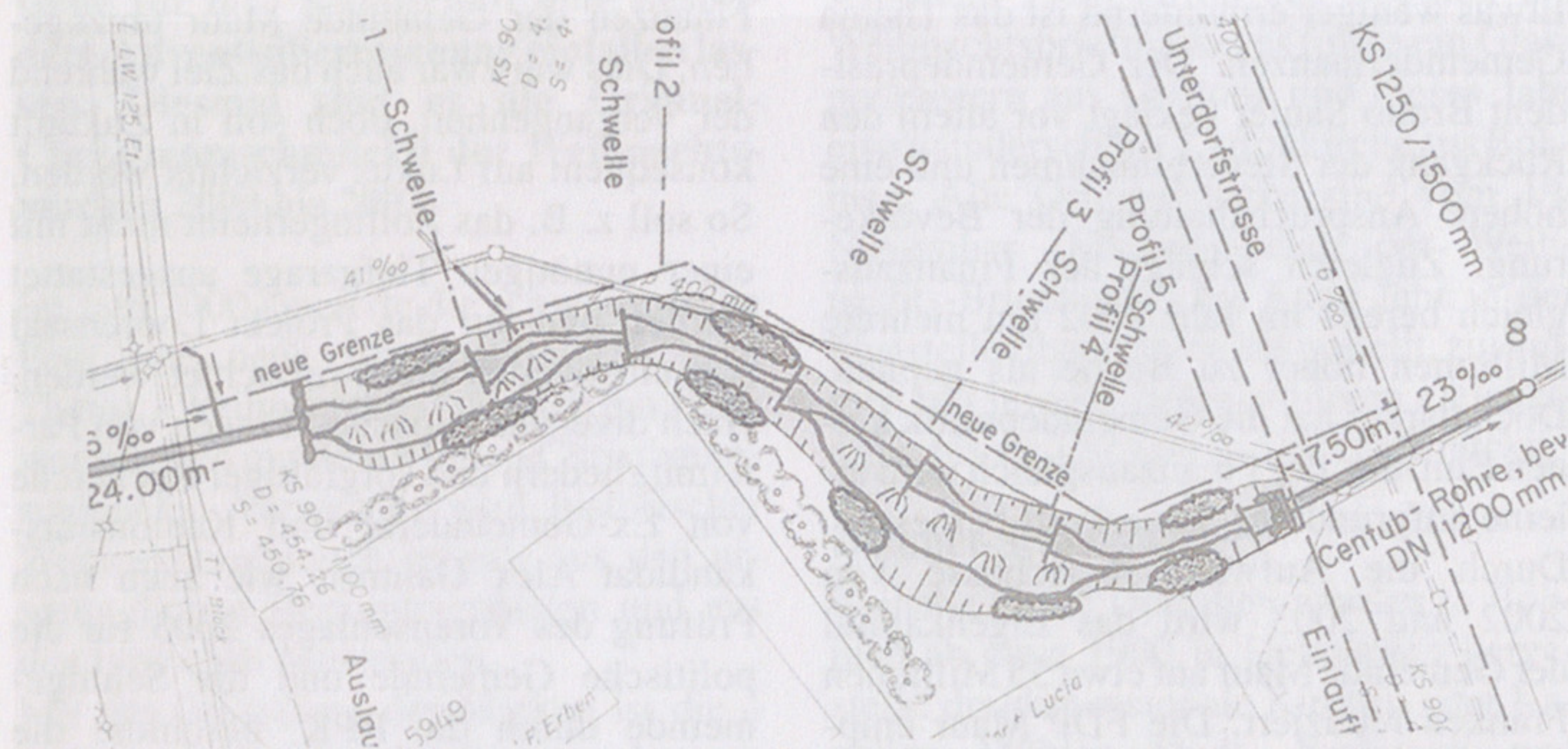
Die Offenlegung des Dattenbachs erfolgt auf rund 70 Metern.
