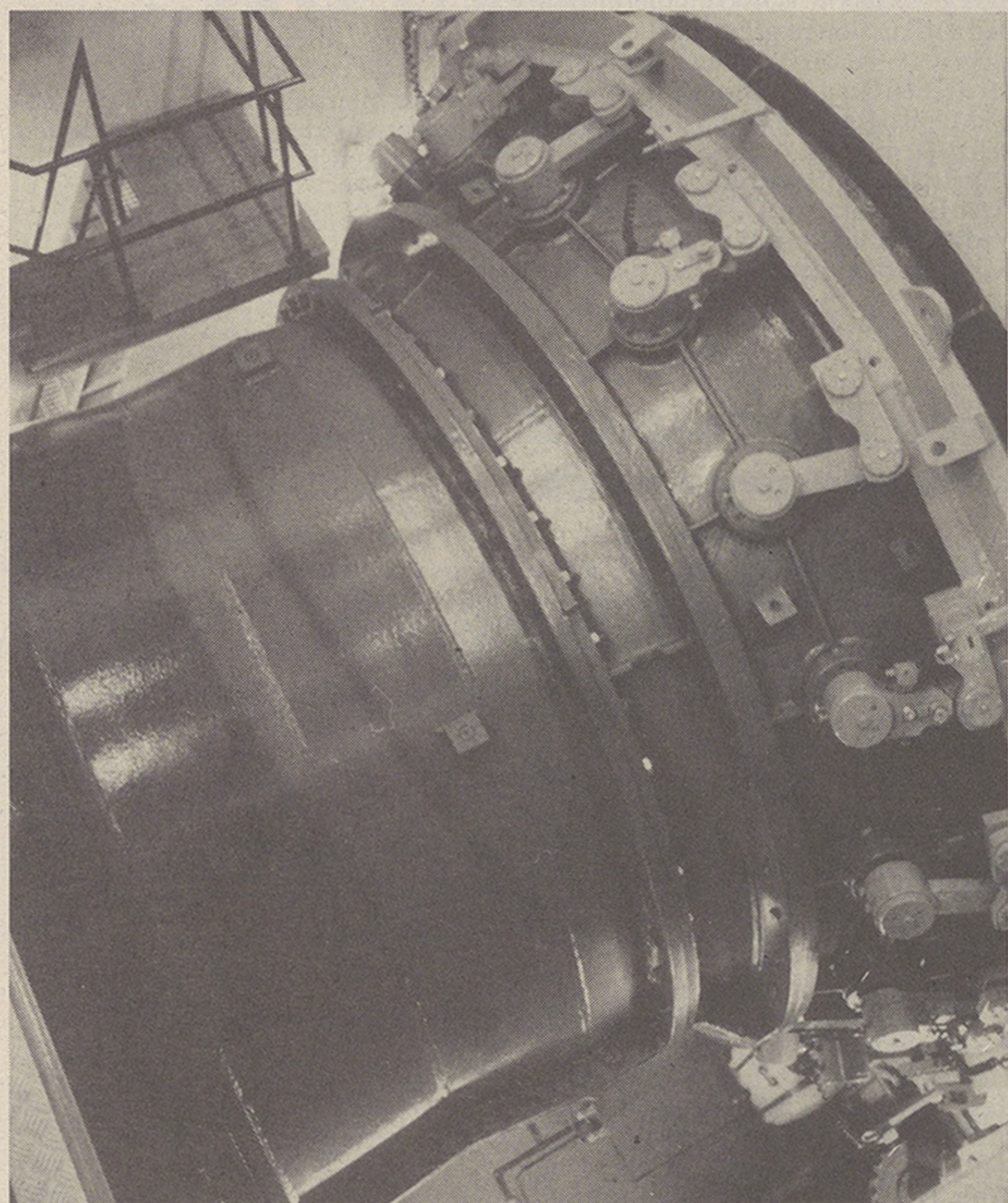
Die neue Rohrturbine im Flusskraftwerk Giessen nutzt Wasserkraft mit modernster Technologie.
