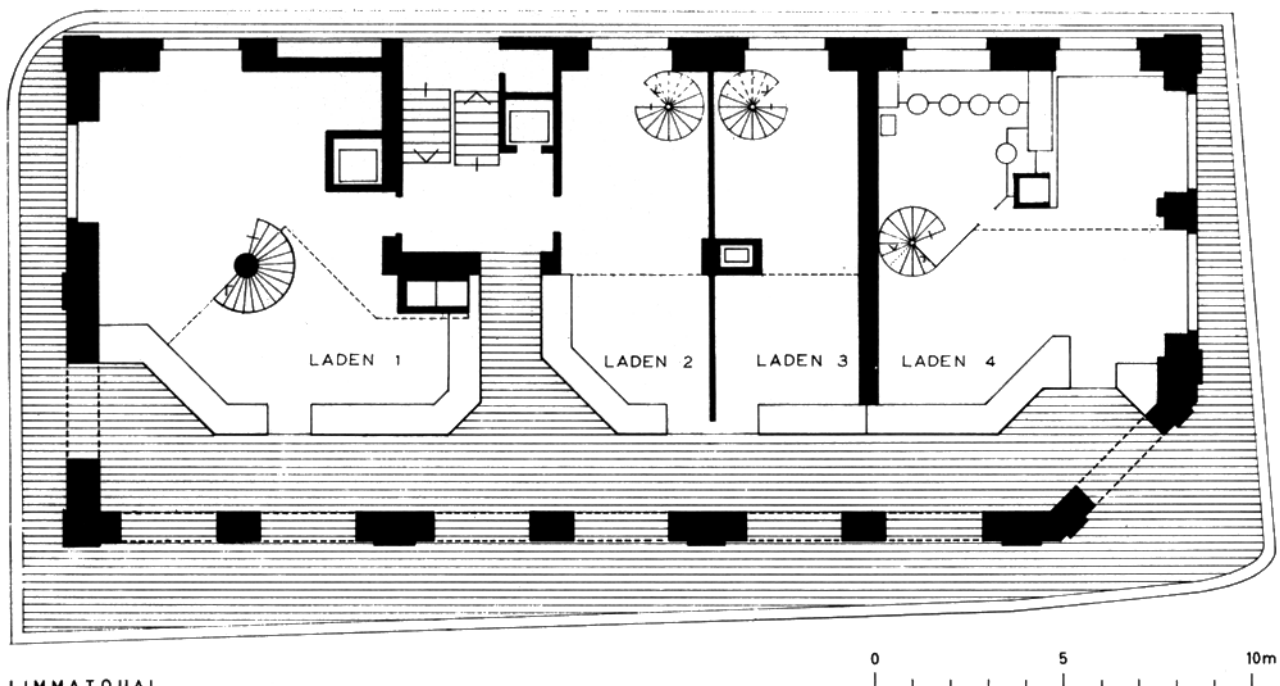
Limmatquai 62. Haus der Museumsgesellschaft. Grundriss des Erdgeschosses.
