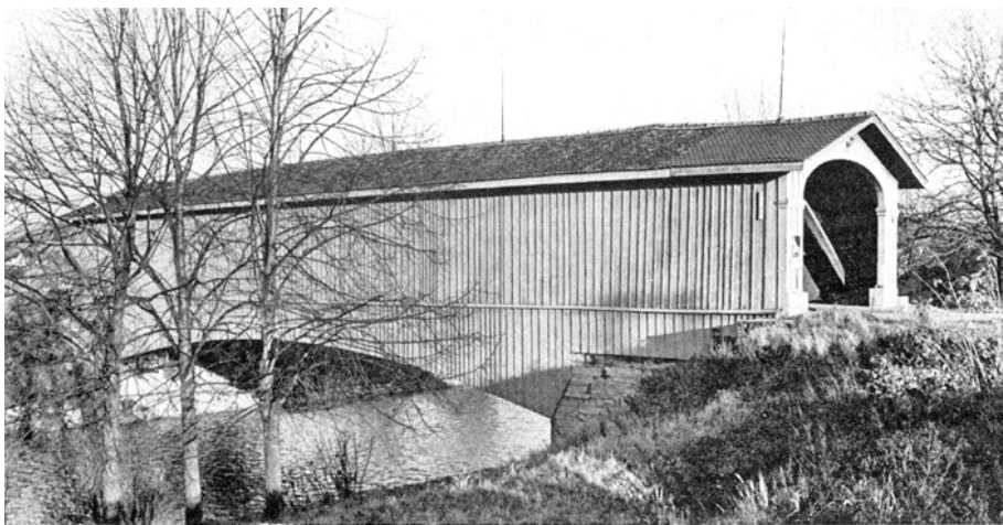
Neftenbach. Gedeckte Brücke im Mittleren Bruni (bei Pfungen).
