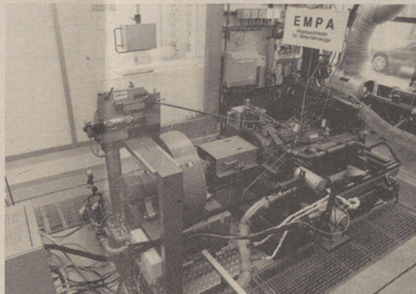
Dieser Dieselmotor wurde bei der EMPA in Dübendorf mit vier verschiedenen Treibstoffen getestet. Seit Sommer 1991 verkehren in der Stadt Zürich mehrere Busse mit diesem Motorentyp.
