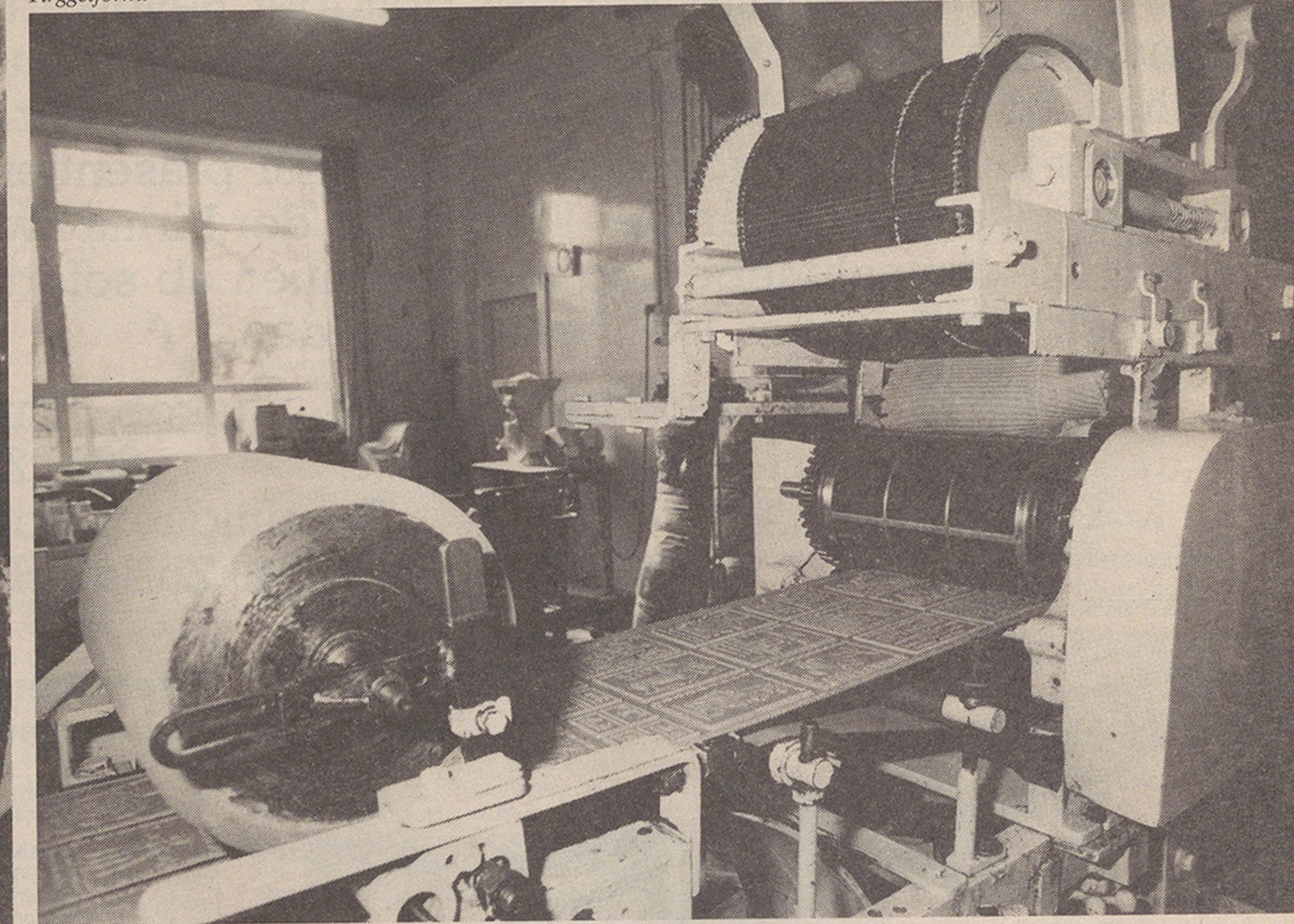
Der noch warme Teig kommt in die Gebäckformmaschine, wird mittels zwei vertikalen Walzen zu einer hauchdünnen Masse ausgewalzt (oben rechts) und erhält durch die Prägewalze (rechts) und der anschliessenden Gummivalze (links) die Tirtgelform.
