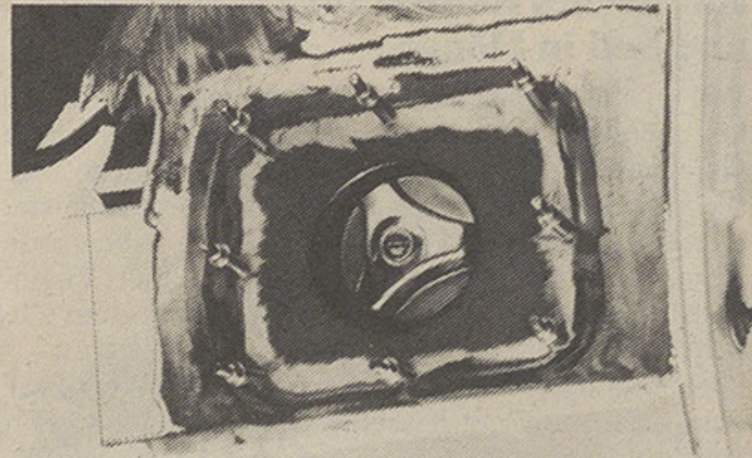
Die neue Carrosserie-Technik «Kleben statt Schweissen» angewandt z.B. bei der Reparatur eines Tankneinfüllstutzen. (Photo Würth AG)
