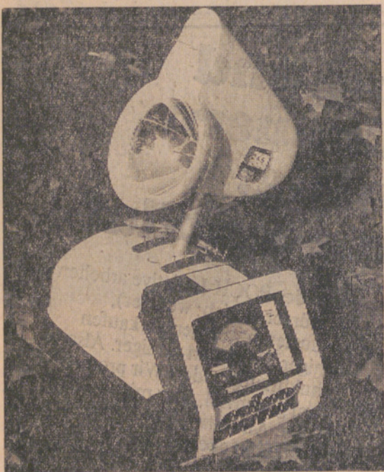
Das Sonnenbrand-Warngerät von Wolfgang Bacsa, Binz, erhielt den 2. Preis im WWF-Jugendwettbewerb.
