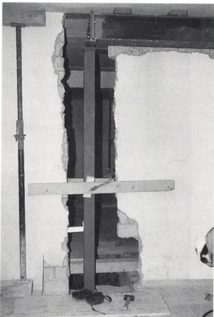
Eine Wandabfangung unter dem Wohnheim: Wandschlitz, neue Stütze mit Abfangträgern.
