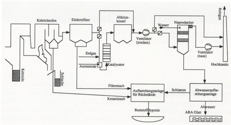
Kehrichtverbrennung mit Rauchgasreinigung nach dem Nass-Prinzip. Die neuen Anlagenteile (rechts) nehmen mehr als die Hälfte des Schemas ein – sie bringen aber auch eine mindestens 10-fache Verbesserung der Abluftqualität.
