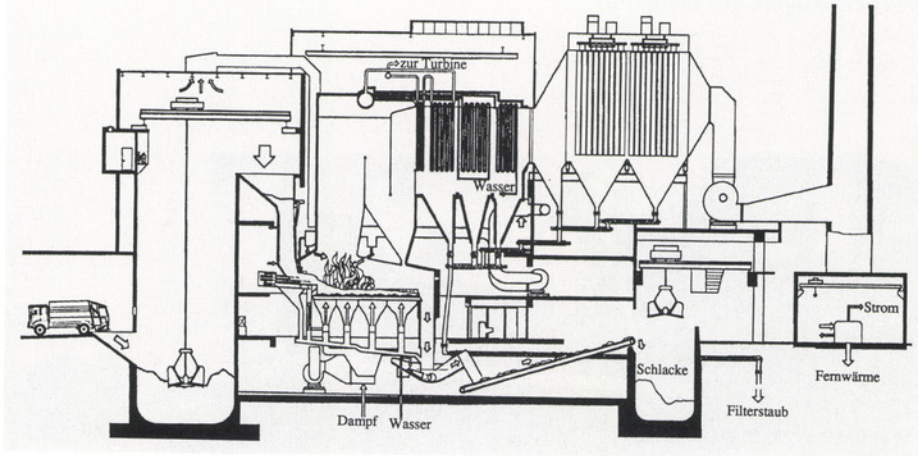
Schnitt durch die Kehrichtverbrennungsanlage Hagenholz (Zustand 1992). Man erkennt v. l. n. r. den Kehrichtschacht, einen Verbrennungsofen, das Röhrensystem für die Dampferzeugung, einen Elektrofilter, die separate Sammlung von Schlacke und Filterstaub, die Nutzung des Dampfes und darüber das Hochkamin.
