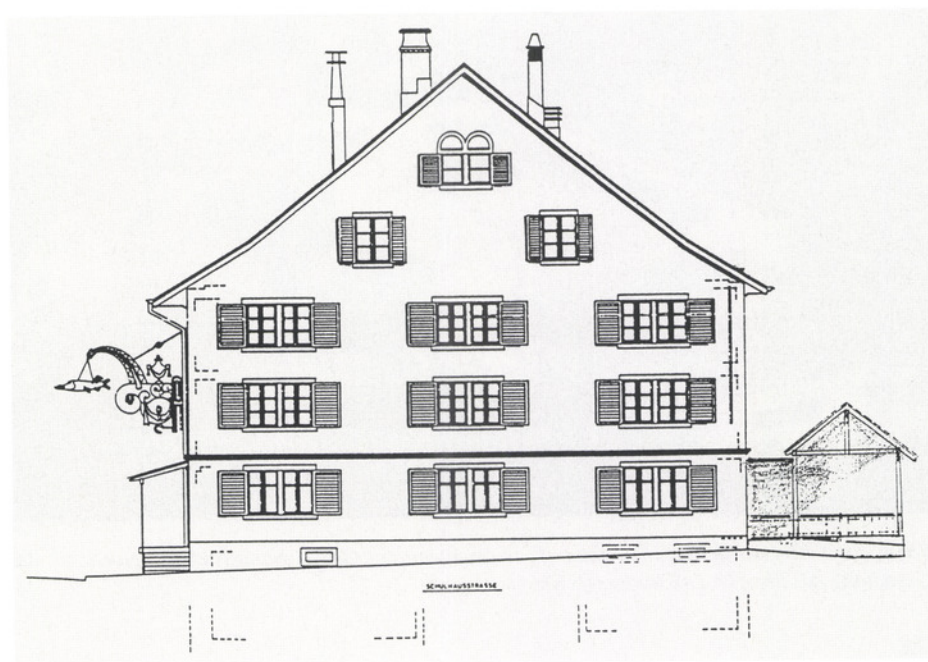
Südwest-Fassade des «Hecht», eine Zeichnung aus dem «Projekt 1992». Deutlich ist der hofseitige Anbau zu erkennen.
