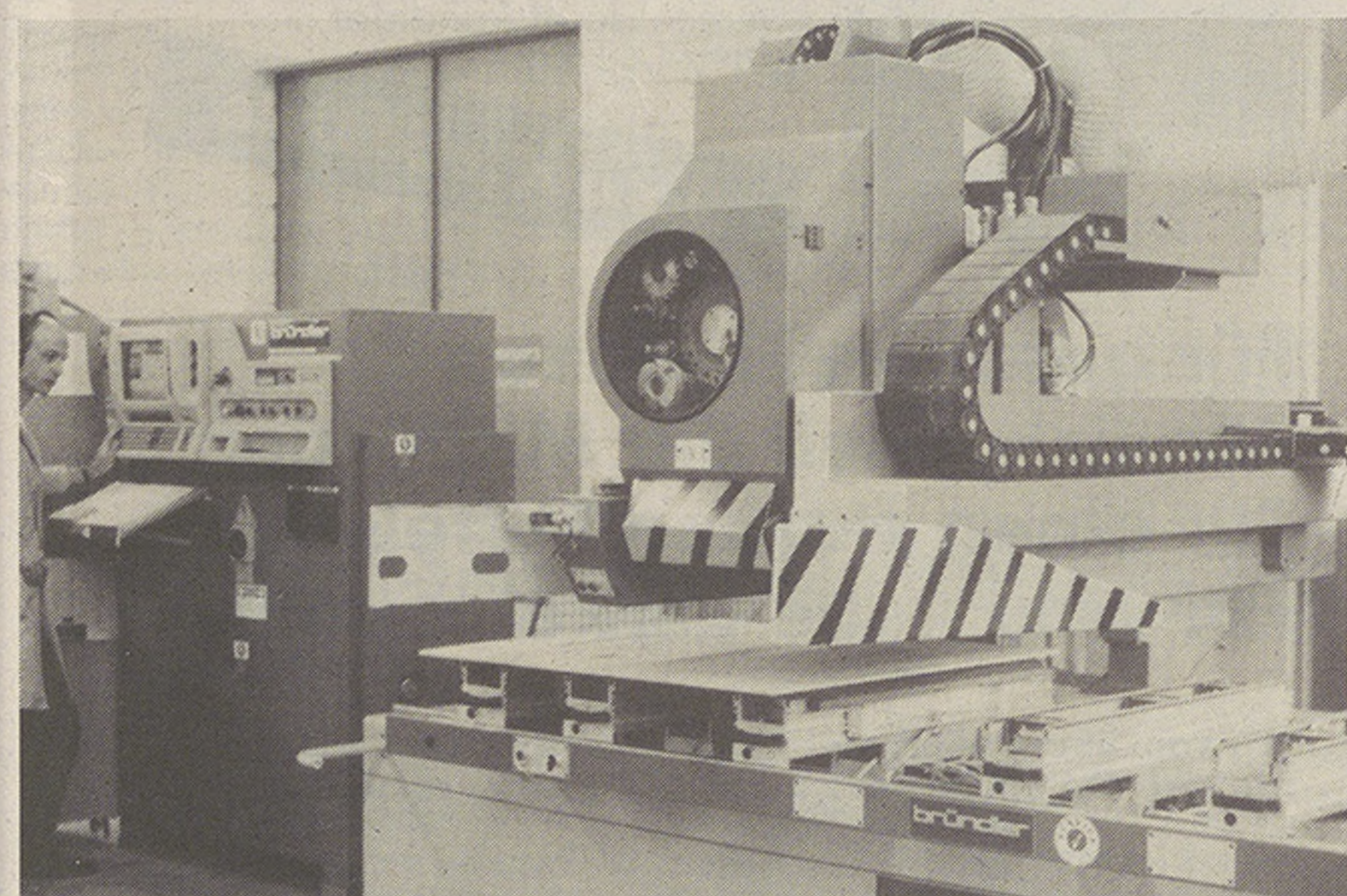
CNC-gesteuerter Fräs- und Bohrautomat, bestückt mit 32 Werkzeugen
