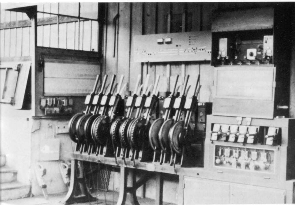
Das Stellwerk mit der Geleisetafel
