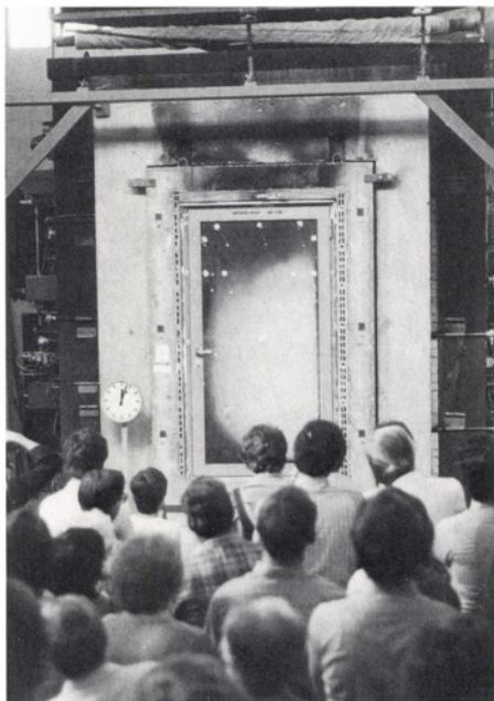
Feuerprobe – ein Test für die Feuerfestigkeit
