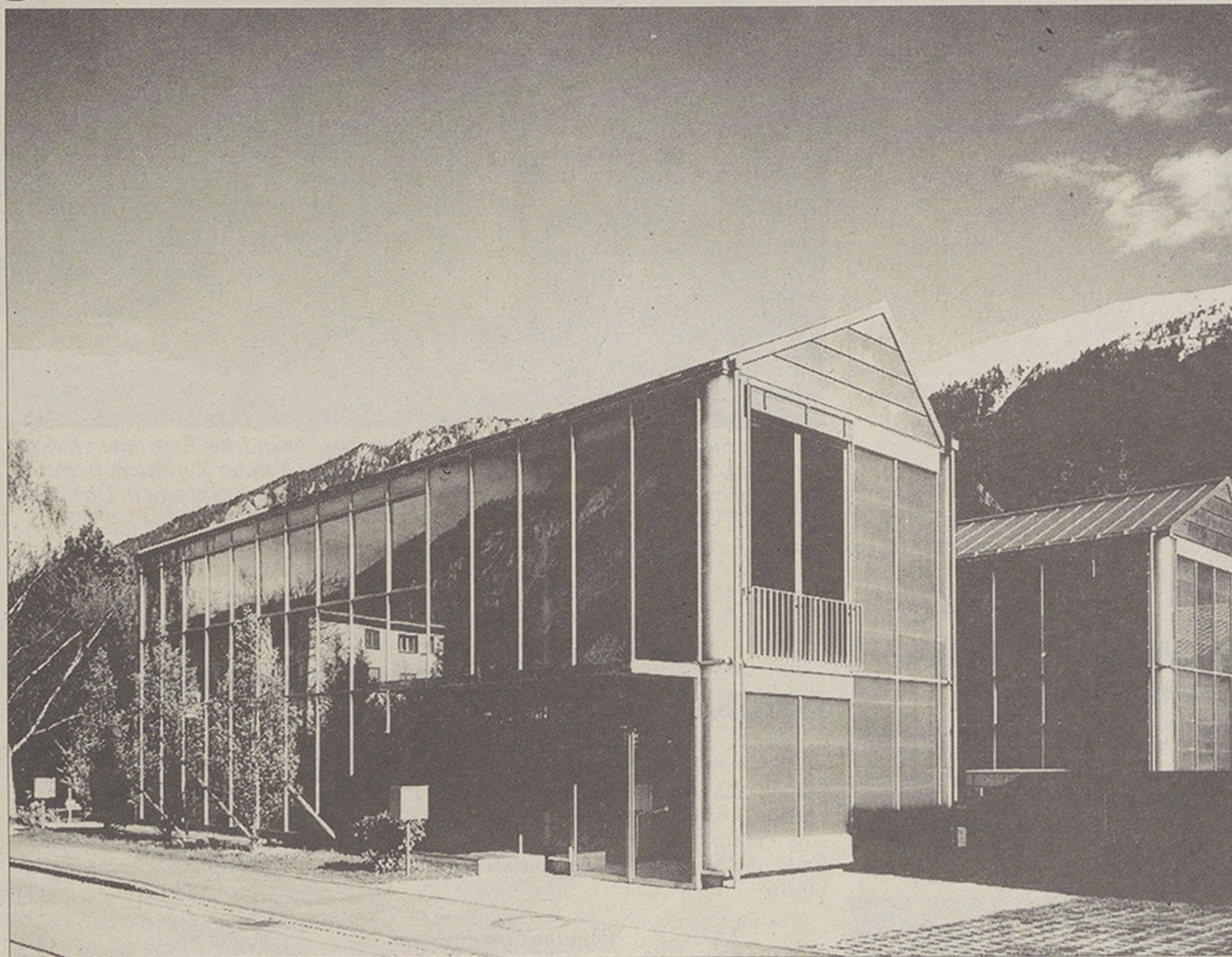
Die konsequente Sonnenenergienutzung bestimmt hier die Architektur: Dietrich Schwarz baut Häuser mit Wänden, die bei Bedarf heizen können und Dächern, die warmes Wasser und Strom produzieren. (Bild Reto Führer)
