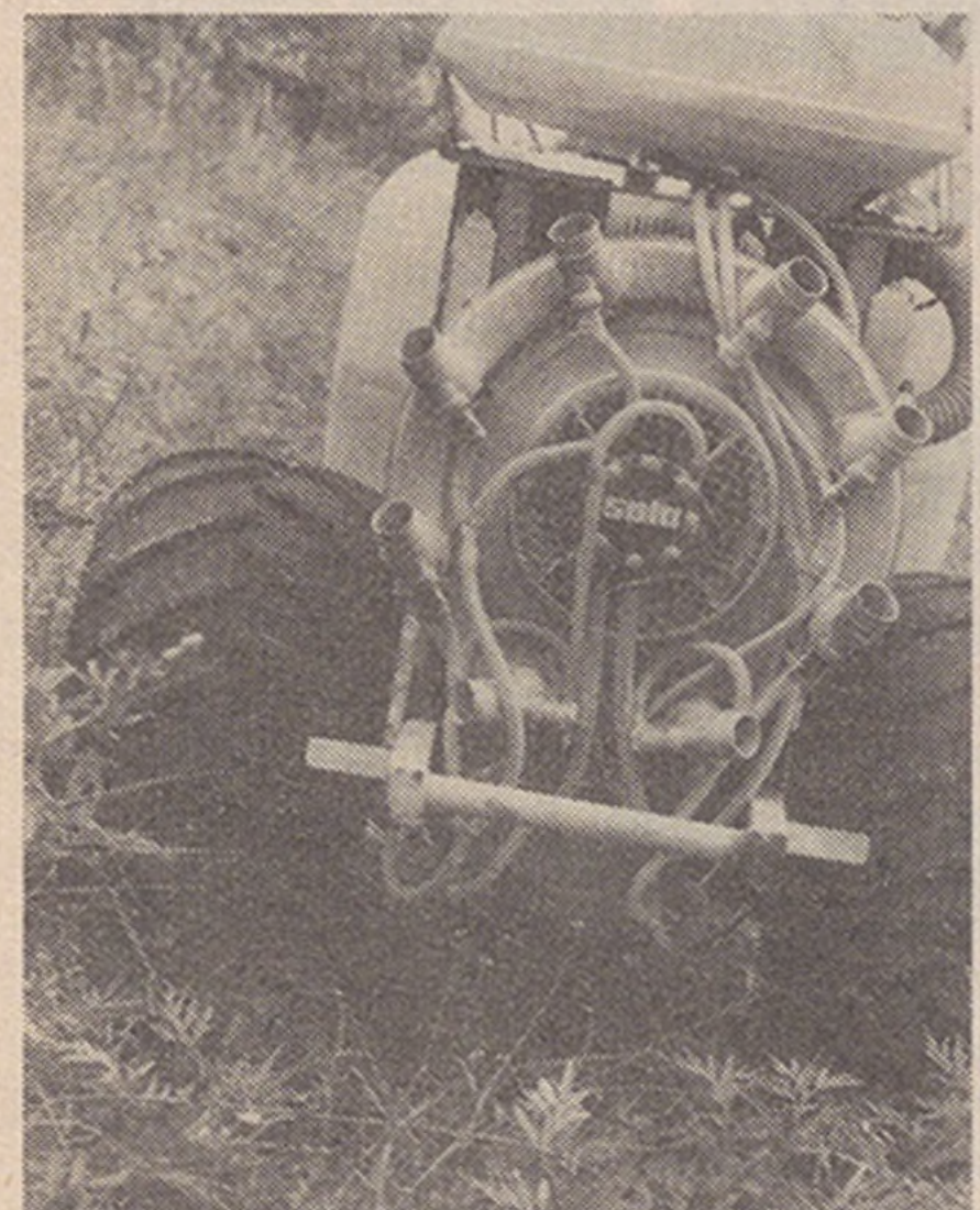
Dieses Maschinenungeheuer kommt auf leisen, breiten Sohlen. Die sehr breiten Pneus reduzieren den Druck auf den Boden, der locker sein soll im Rebberg. Das Ungeheuer wirkt auch deshalb bedrohlich weil es Mittel, nicht von der «Grünen Wiese», zerstäubt... wenn einmal nötig. Diesbezüglich übt man heute äusserste Zurückhaltung. Dasselbe gilt für die künstliche Düngung. Während der Ostschweizer Rebbaubauer mit vierzig bis fünfzig Kilogramm pro Hektare eine gute Qualität anstrebt, wird in Deutschland teilweise heute noch zirka 400 kg pro ha empfohlen.
