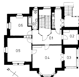
Erdgeschoss
