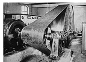
Vorwerk- und Turbinengebäude Vers. Nr. 30. Kraftübertragung von der Turbine auf den 500-Volt-Generator mittels Schwungrad und vernietetem Antriebsriemen. Zustand 1979. Bild aus Dok. 21.
