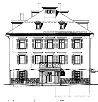
Villa «Neuhof», Aufriss der Hauptfassade. Zeichnung: Architekturbüro Heinrich Th. Uster AG, Wädenswil/Egg, 1993, Mst. 1:100 (verkleinert).
