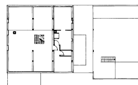
1. Dachgeschoss
