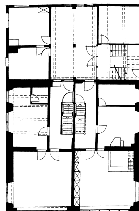
Grundriss des Erdgeschosses nach der Renovation. Zeichnung kantonale Denkmalpflege. Mit breiten Mauern das ursprüngliche Gebäude; Südost-Stube mit grünem Kachelofen. Im nördlichen Anbau von 1802 das neue Treppenhaus mit Stahlterasse.
