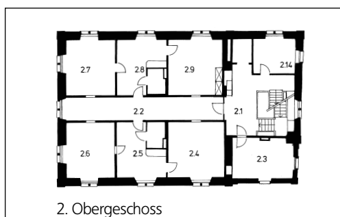
Grundrisse des 1. und 2. Obergeschosses. Zeichnungen kantonale Denkmalpflege. Man beachte die neu eingebauten Nasszellen der Zweizimmer-Appartements (Räume 0.7, 1.5, 1.8, 2.5, 2.8).
