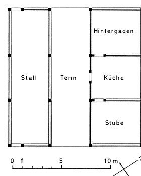
Axonometrie und Grundriss (schematisiert) des Kernbaus von 1536/1545. Zeichnungen 1991 (verkleinert) von Attilio d'Andrea, Architekt, Forch. (Dok. 6)
