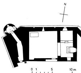
Grundriss der Schlosskapelle Kyburg. Zeichnung kantonale Denkmalpflege. Links das Schiff, rechts unten der Chor, darüber der Nebenchor.
