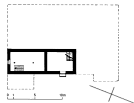
Untergeschoss
