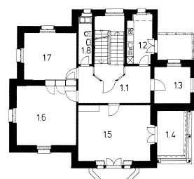
1. Obergeschoss
