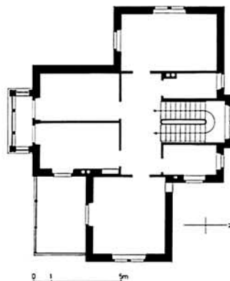
Grundriss des 1. Obergeschosses. Zeichnung kantonale Denkmalpflege. Die Grundrisse sind in allen Geschossen beinahe identisch.
