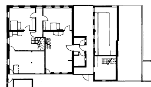
Erdgeschoss
