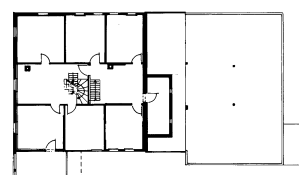
Obergeschoss
