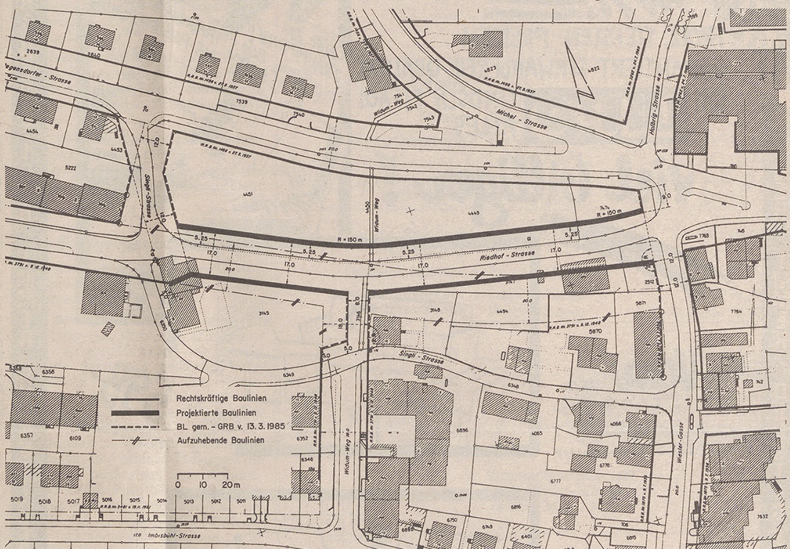
Baulinien-Revision Riedhofstrasse Höngg, abgeändert gemäss Antrag der vorberatenden Kommission des Gemeinderates
