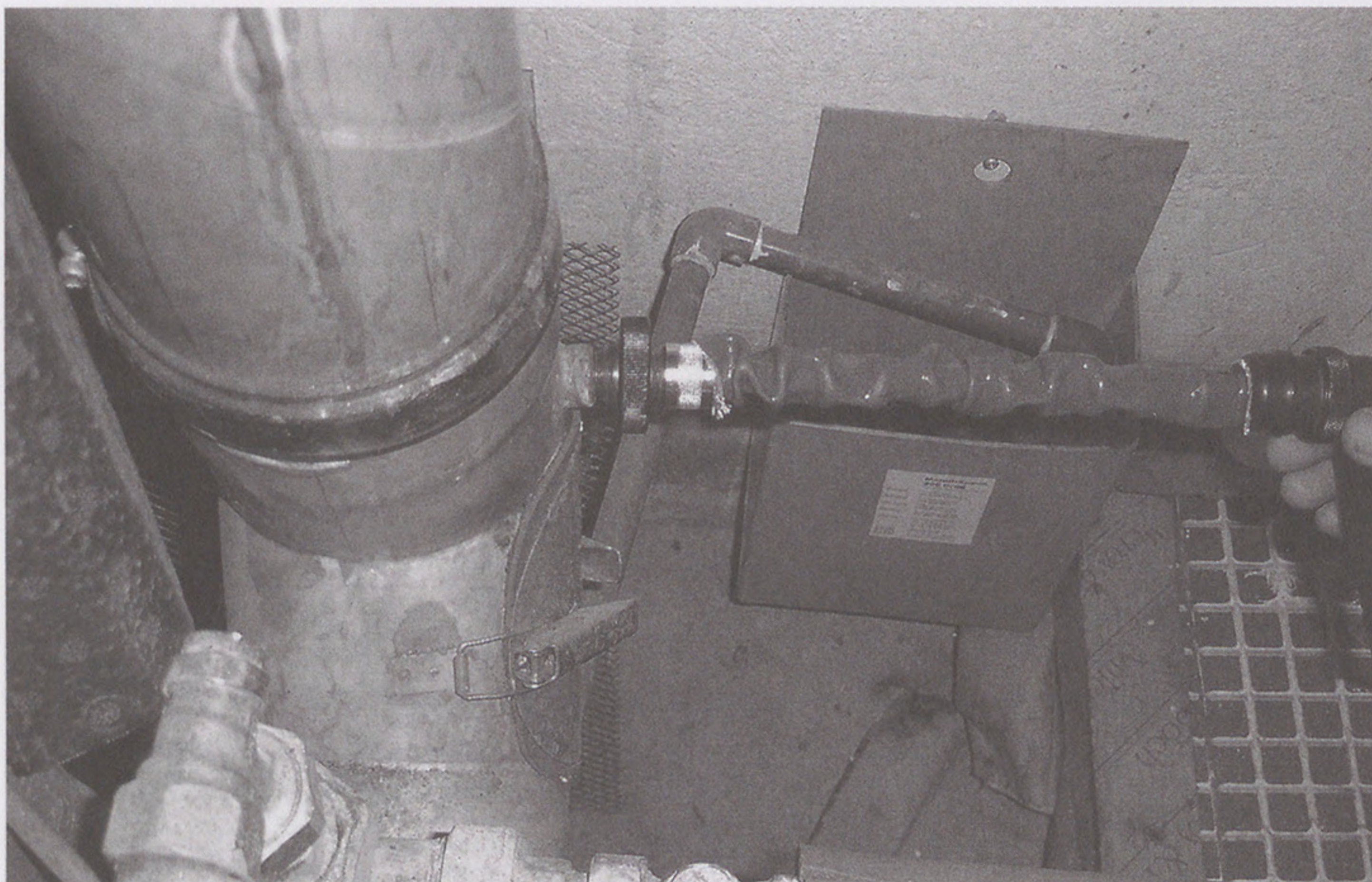
Der rote Peilmessstab wird ins Zubringerrohr geführt und liefert die Messwerte.
