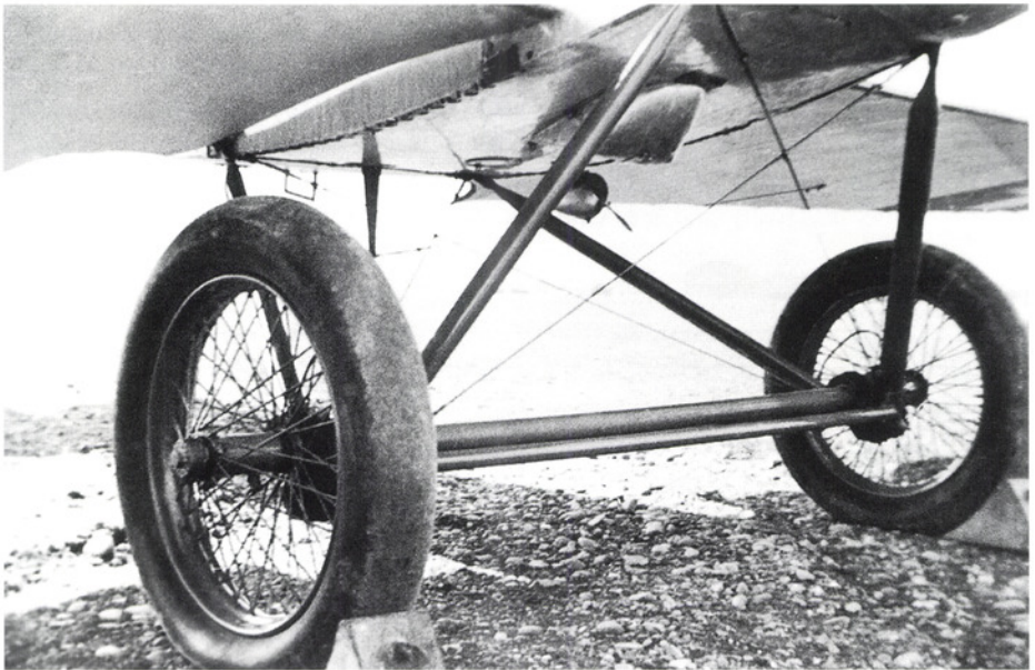
Detailaufnahme eines DH-3: die Räderachse ist mit Gummikabeln festgehalten.
