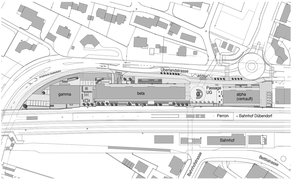
Situationsplan der neuen Überbauung InsiderPark beim Bahnhof. Deutlich sind die engen Platzverhältnisse zu erkennen, die das Planen und Bauen sehr anspruchsvoll machten.
