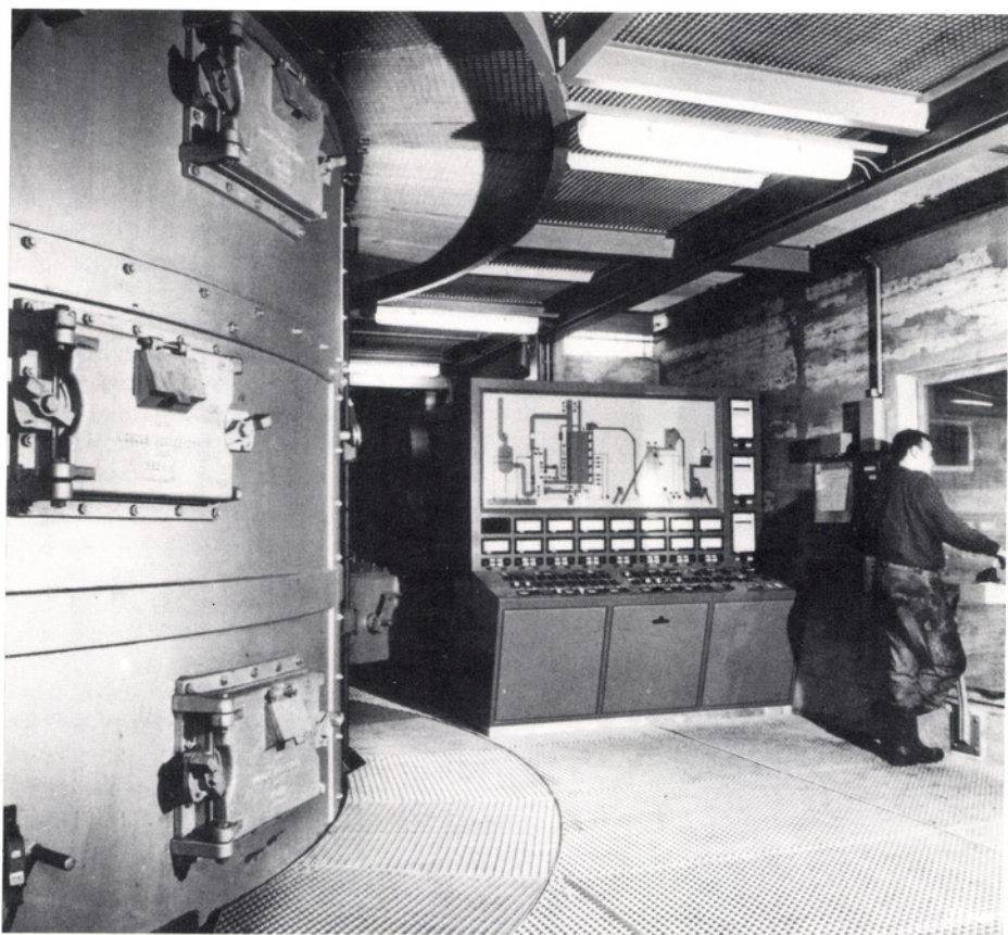
Im Innern der Kehrichtverbrennungsanlage. Links der Ofen und rechts das Kommandopult. Daneben das Beobachtungsfenster zum Kehrichtbunker.
