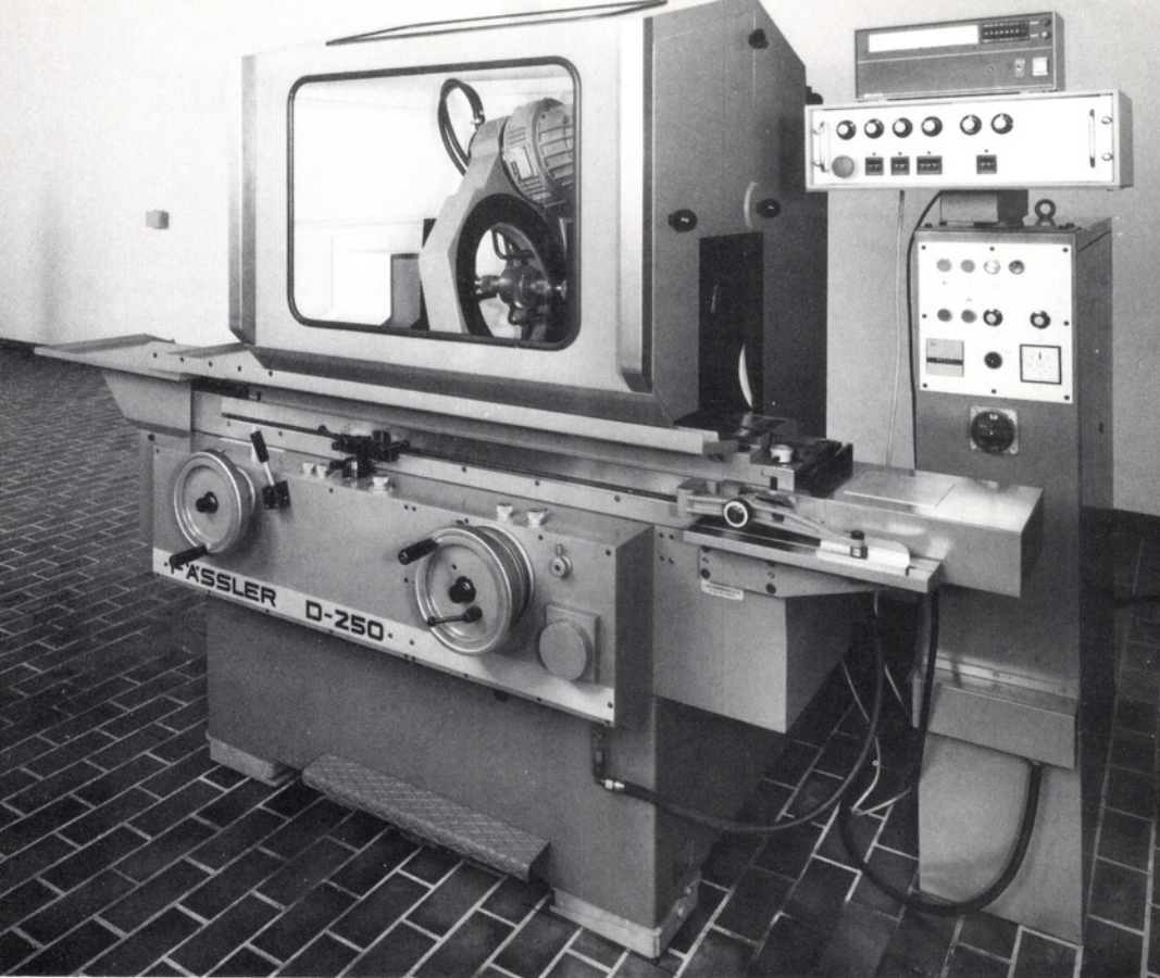
Zahnradhonmaschine (honen = feinschleifen) hergestellt bei der Firma Fässler AG in Dübendorf.
