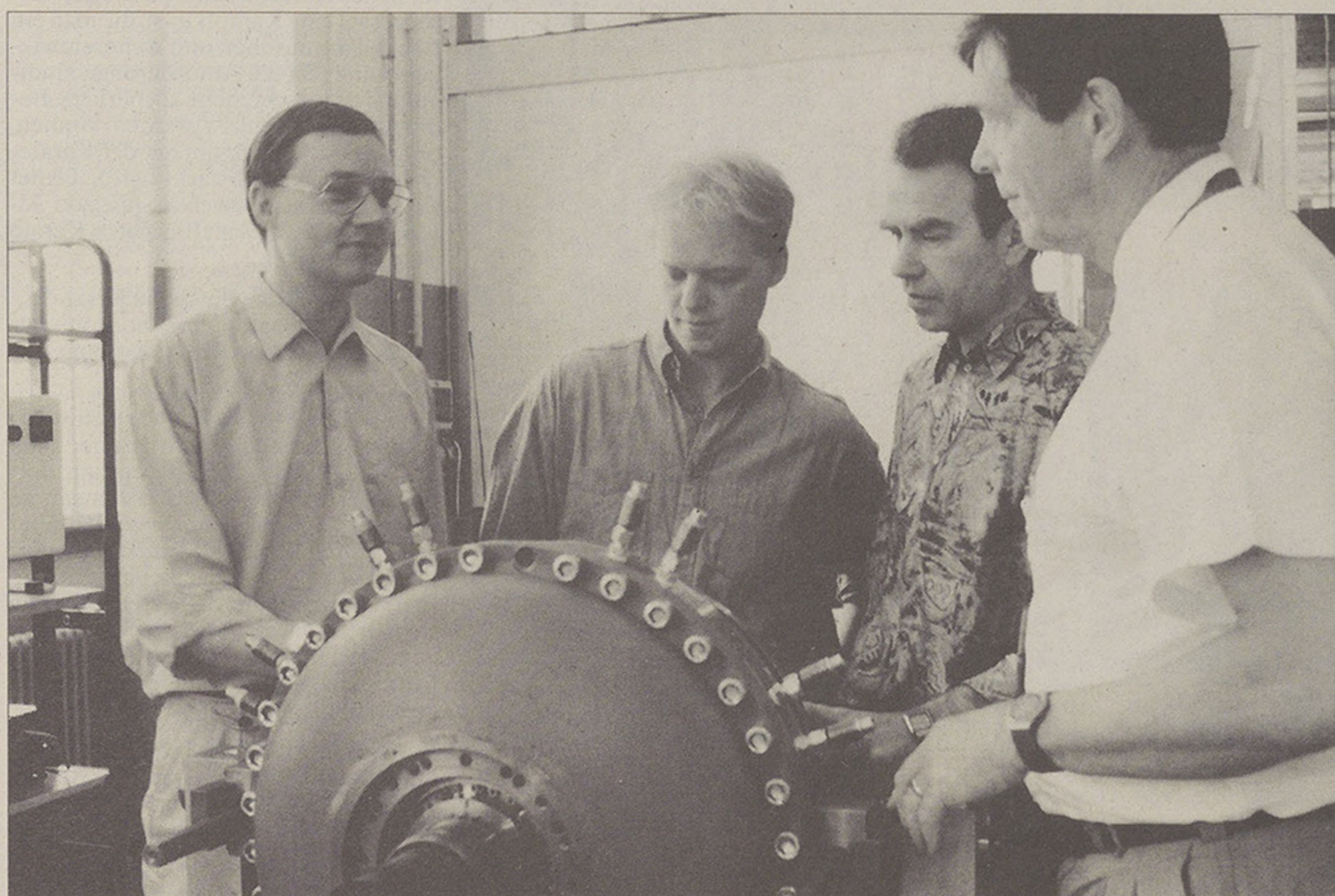
Solche erdgasbefeuerte Stirling-Maschinen zur kombinierten Strom- und Wärmeproduktion könnten künftig in vielen Heizkellern stehen. Die Pilotanlage liefert gute Resultate. (Bilder Nadja Athanasiou)
