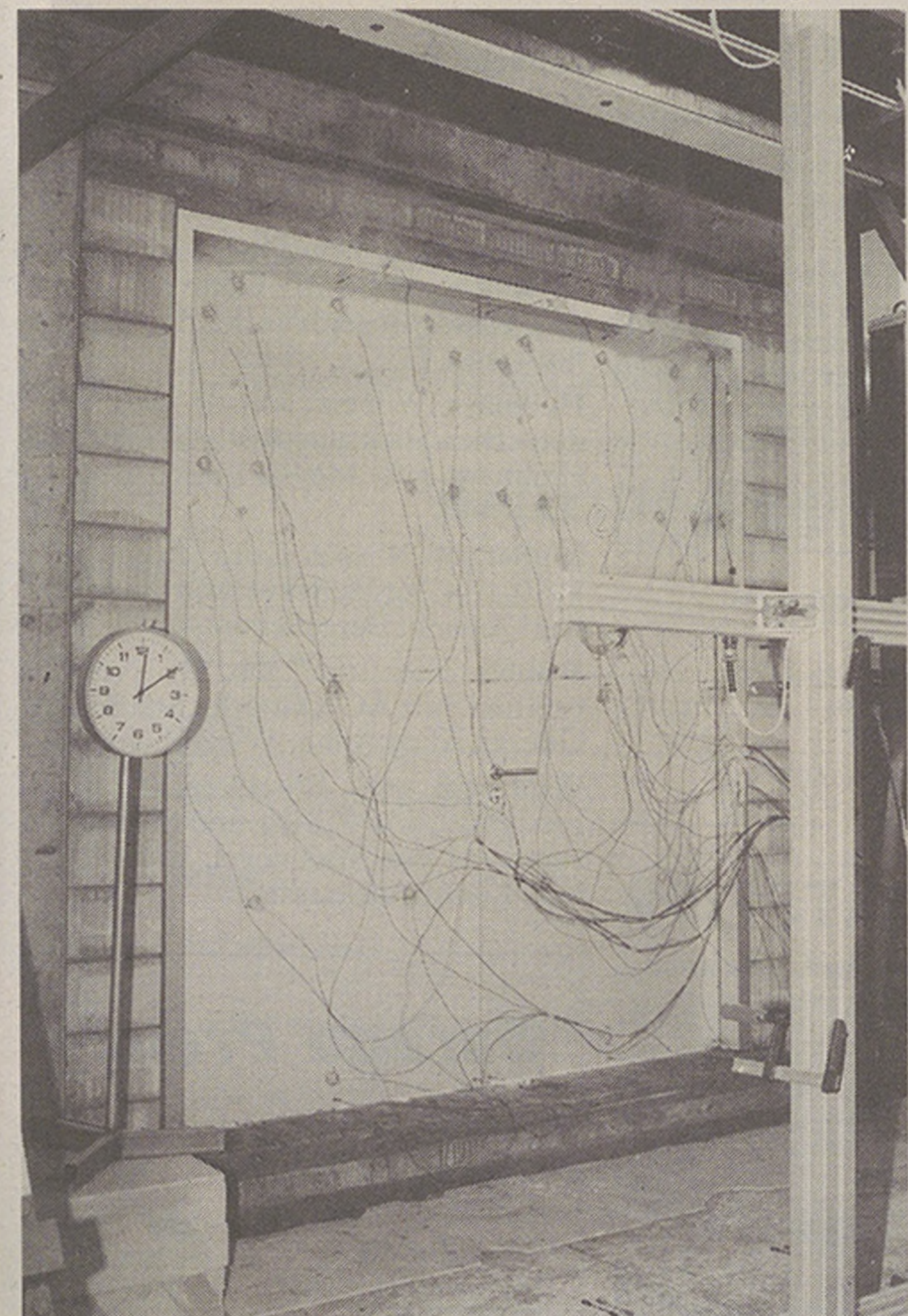
Prüfungsanordnungen mit Messpunkten und Uhr. Sie zeigt, wie lange die Türe der Brandeinwirkung zu widerstehen vermag.
