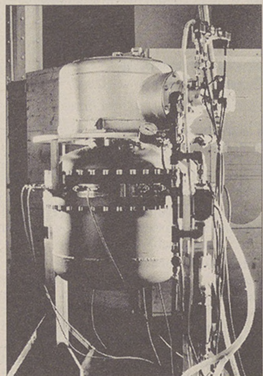
Solche erdgasbefeuerte Stirling-Maschinen zur kombinierten Strom- und Wärmeproduktion könnten künftig in vielen Heizkellern stehen. Die Pilotanlage liefert gute Resultate. (Bilder Nadja Athanasiou)
