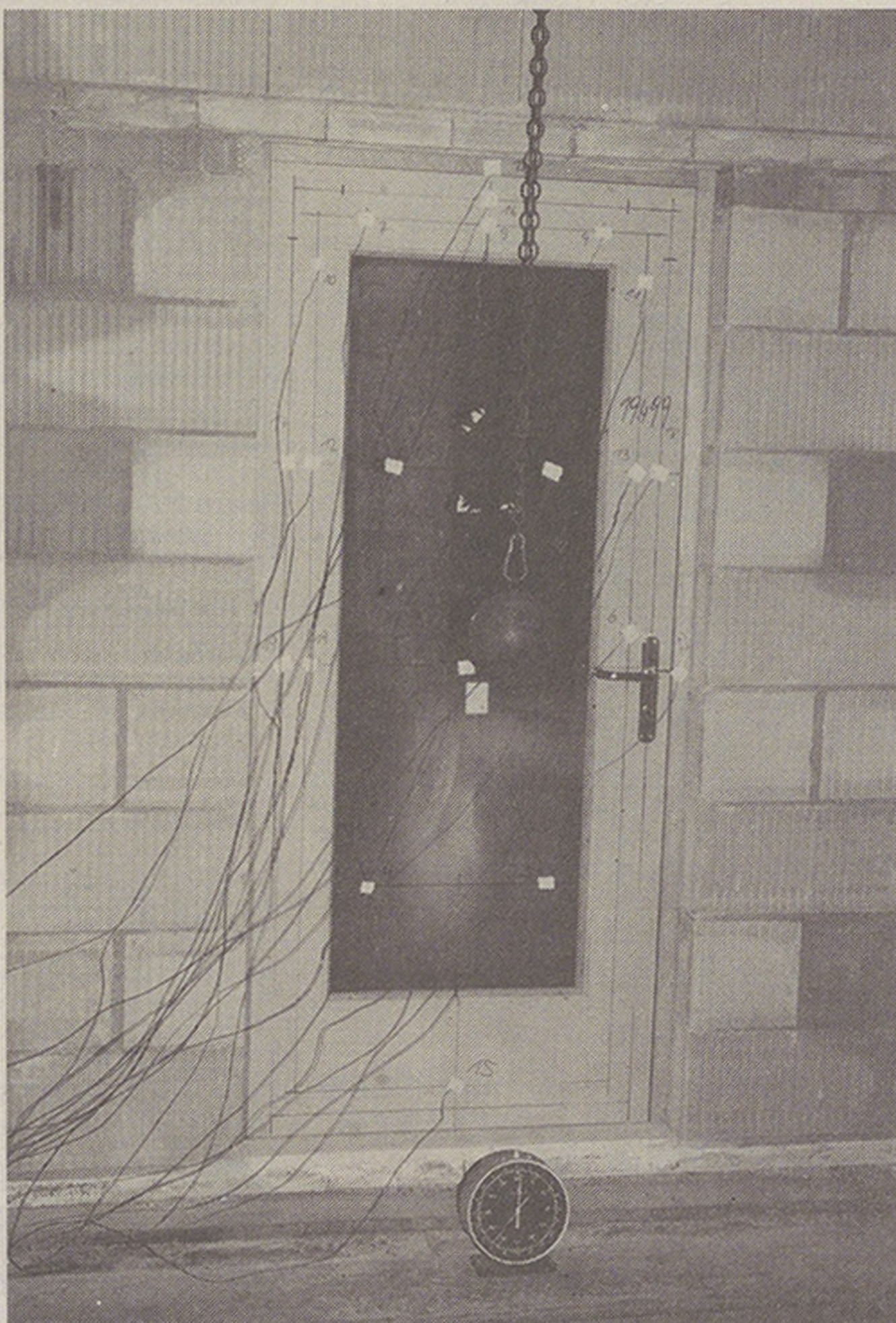
Holz/Glas-Brandschutztüre T30 während des EMPA-Tests.
