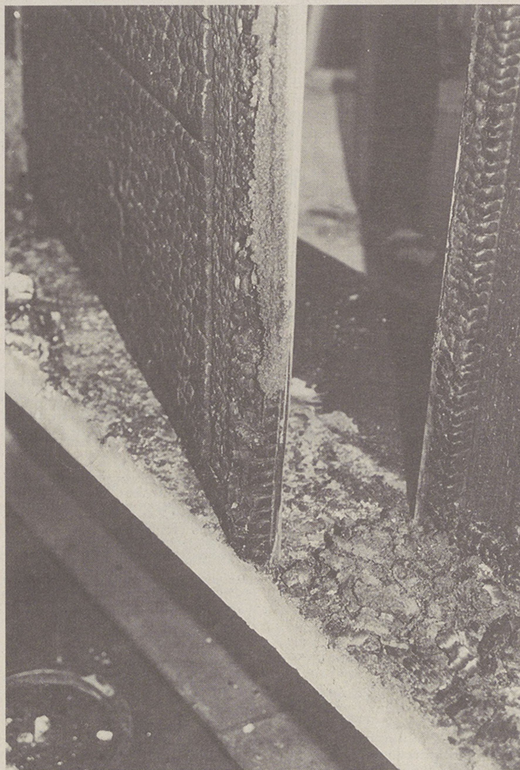
Test bestanden: Innenansicht der Türe nach dreissig Minuten Brandeinwirkung.
