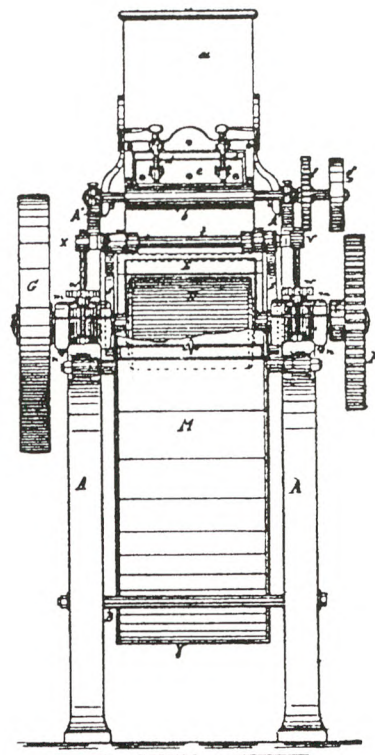
Pläne des von Friedrich Wegmann entwickelten Walzenstuhls.
