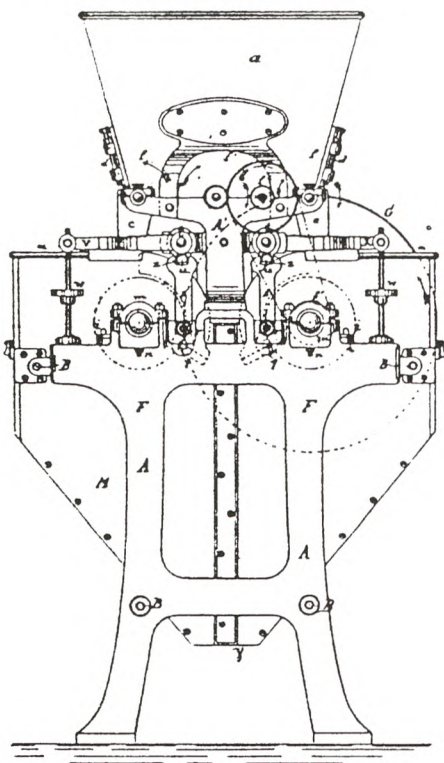
Pläne des von Friedrich Wegmann entwickelten Walzenstuhls.
