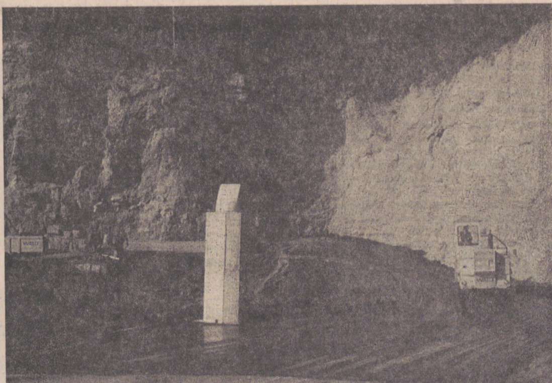
L.R. Mitte Oktober ist in der Chalen der bituminöse Dichtungsbelaag in der Sohle der zukünftigen Multikomponentendeponie eingebaut worden. Der «Turm» in der Bildmitte ist der Sammelschacht für die Abwässer aus der Deponie. (Foto: Ing. G. Mugglin)
