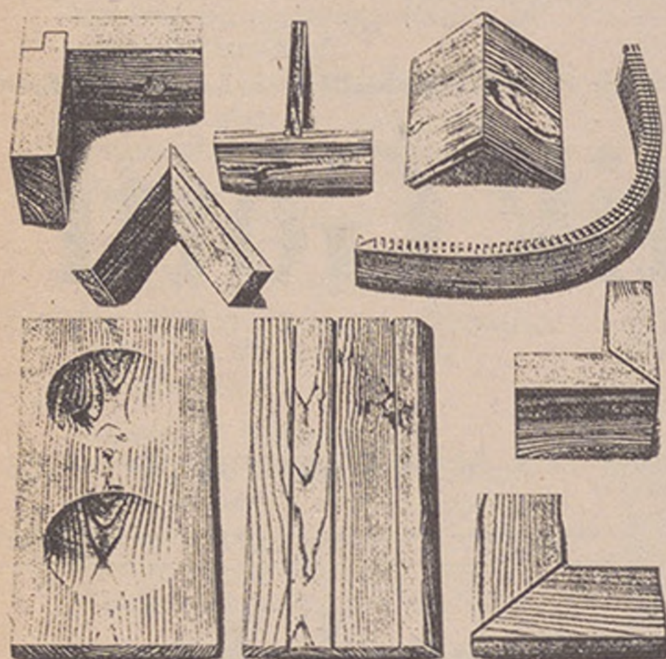
Beispiele der Arbeitsmöglichkeiten mit einem normalen Sägeblatt
