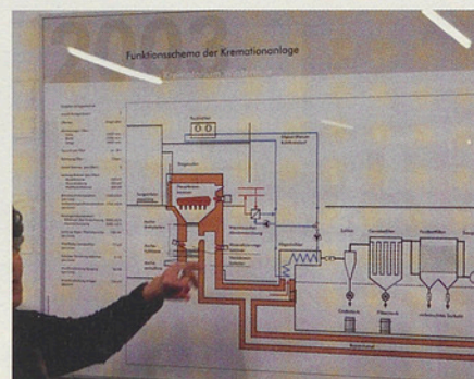
Funktionsschema der Krematoriumsanlage
