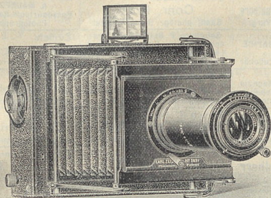
Minimum-Palms 9 \times 12 mit Tessar 1/6 . 3 f = 145 mm und Teleansatz I, fertig zur Teleaufnahme.
