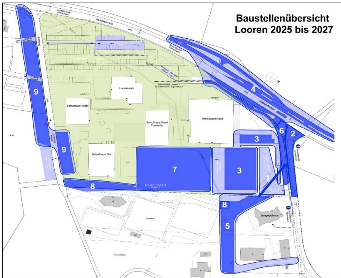
Eine Übersicht über die verschiedenen geplanten Bauvorhaben: 1 Höherlegung Haldenbach; 2 Sanierung Loorenstrasse; 3 Bevölkerungsschutzgebäude; 4 Projekt Aeschstrasse; 5,8,9 Revitalisierung Rausen- und Haldenbach; 6 Trottoir Loorenstrasse; 7 Kunstrasenspielfeld.
