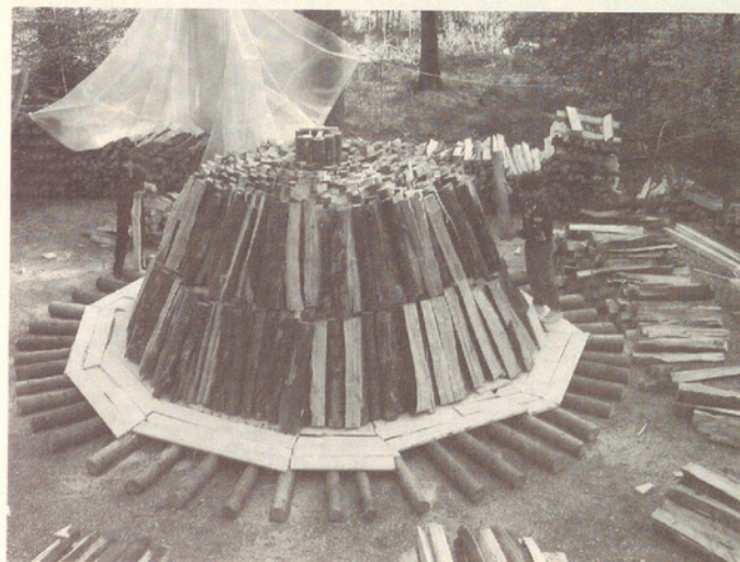
Meileraufbau auf dem Bretterrost
