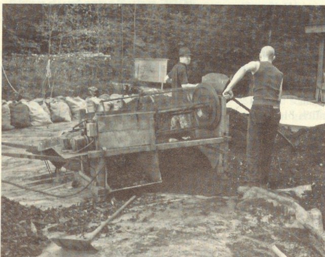
Nach Grösse sortierte Kohle wird abgepackt
