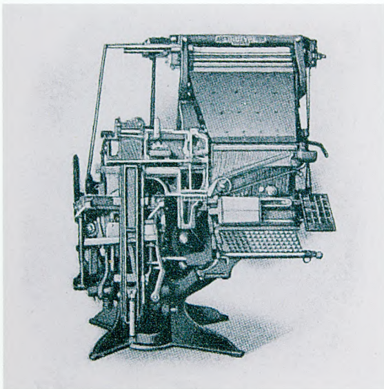
Zeitungsdruckmaschine von 1912.
