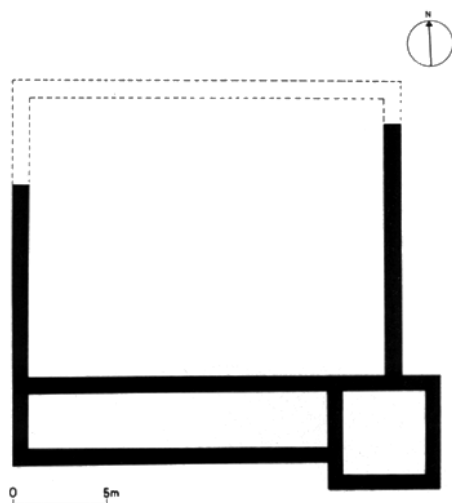
Zell – Kirche. Grundriss des römischen Herrenhauses, teilweise ergänzt.
