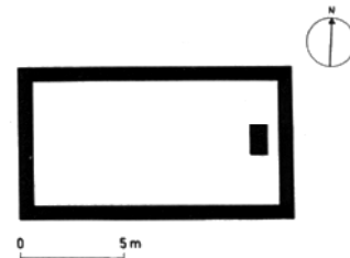
Zell – Kirche. Grundriss der Saalkirche des 9./10. Jahrhunderts.
