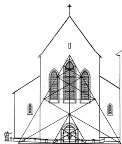
Proportionendreieck an der Westfassade.
