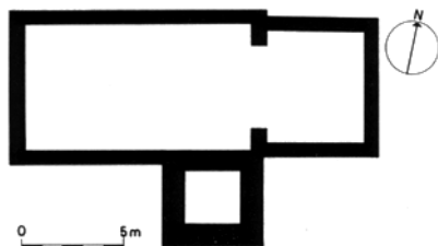
Mönchaltorf – Kirche. Grundriss der romanischen Kirche nach dem Turmbau.
