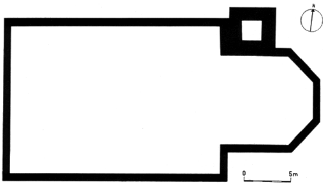
Hombrechtikon – Reformierte Kirche. Grundriss der heutigen Kirche mit dem gotischen Turm.
