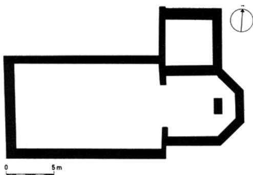
Zell – Kirche. Grundriss der heutigen, das heisst spätgotischen Kirche.
