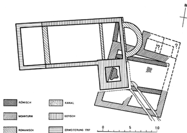
Elsau – Kirche. Baugeschichtliche Untersuchungen 1959: Bauetappenplan 1 : 250.
