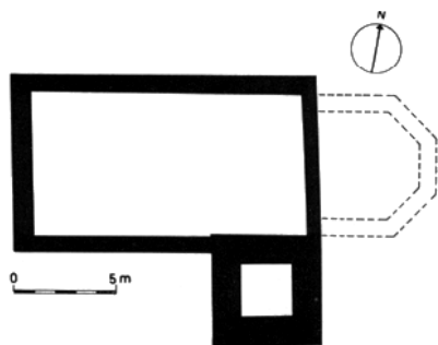
Elsau – Kirche. Grundriss der gotischen Kirche mit dem geplanten polygonalen Chor.
