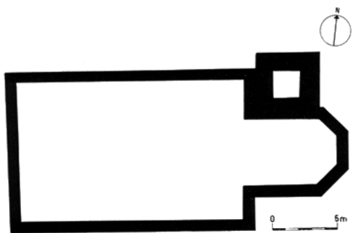
Hombrechtikon – Reformierte Kirche. Grundriss der gotischen Kirche nach dem Turmbau.
