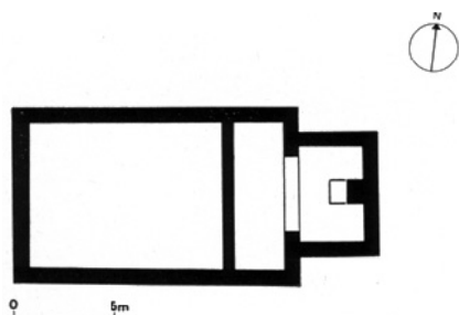
Hombrechtikon – Reformierte Kirche. Grundriss der romanischen Kapelle.
