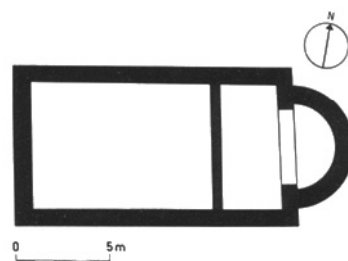
Elsau — Kirche. Grundriss der romanischen Kirche.
