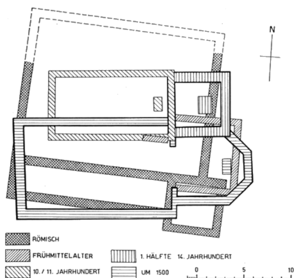
Zell – Kirche. Baugeschichtliche Untersuchungen. 1958/59: Baustapppenplan 1 : 250.
