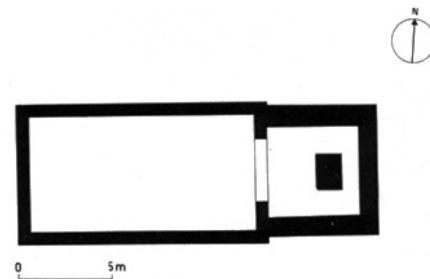
Zell – Kirche. Grundriss der Kirche des 14. Jahrhunderts mit dem Turmchor beziehungsweise Chorturm.
