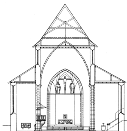
Augustinerkirche 1 : 400. Veränderung der Kirchendecke.
