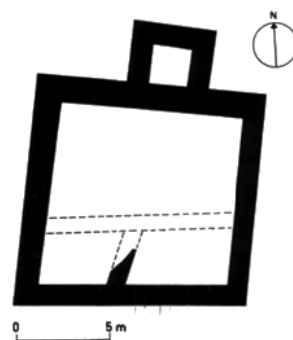
Elsau – Kirche. Grundriss des Wohnturmes mit rekonstruiertem Anbau.
