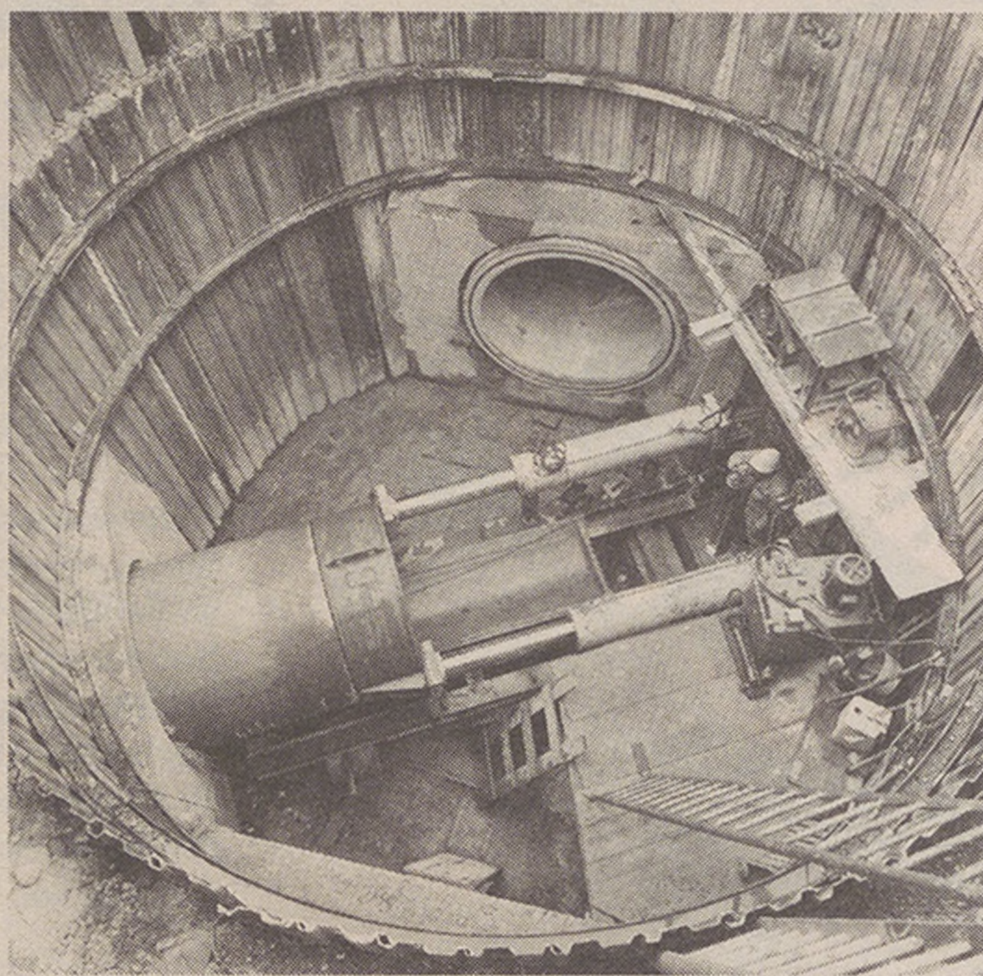
Hydraulische Pressvortriebs-Anlage
