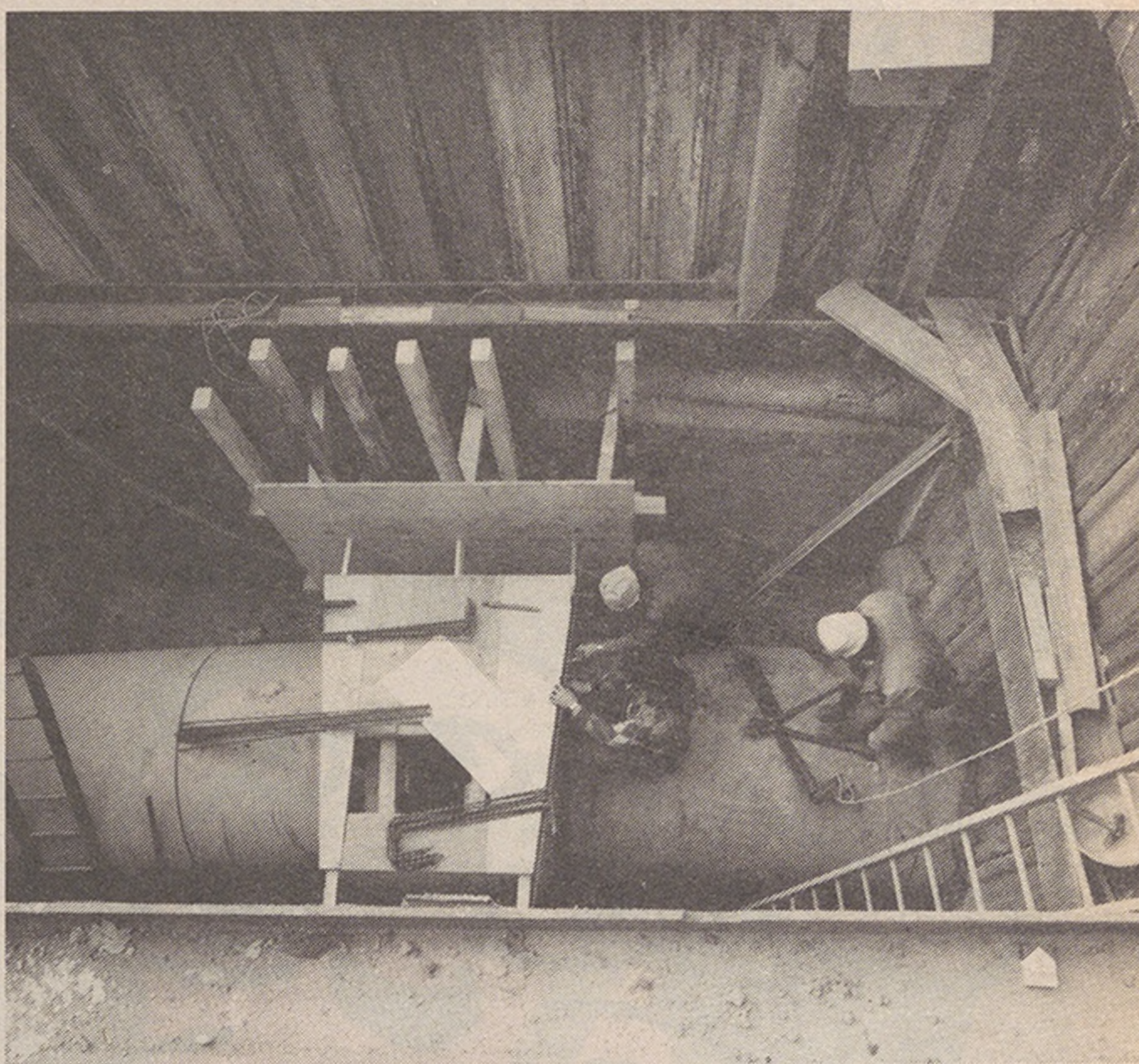
Spezialbauwerke für die Kanalisation, z. B. ein 10 Meter tiefer Absturzschaft
