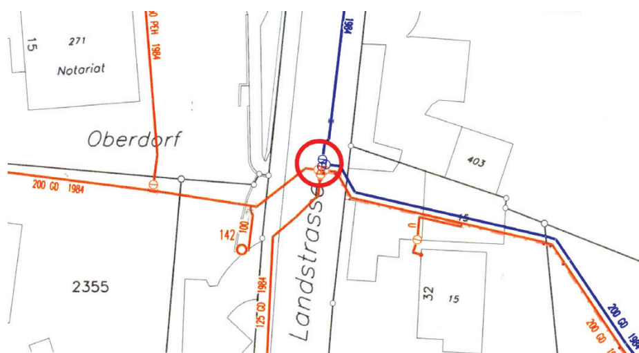
Standort Schacht in der unteren Druckzone
