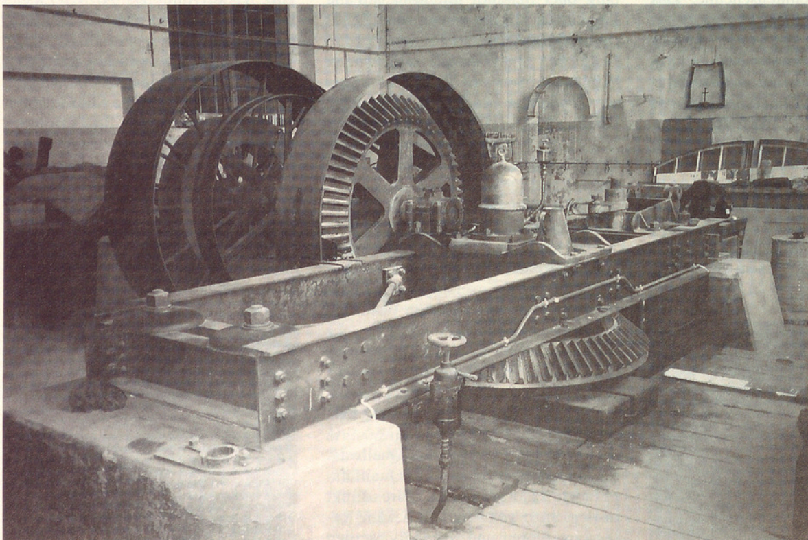
Die vertikalachsiges Turbine und das Holz- und Eisengetriebe von 1882 der Kraftzentrale Schönenberg TG.
