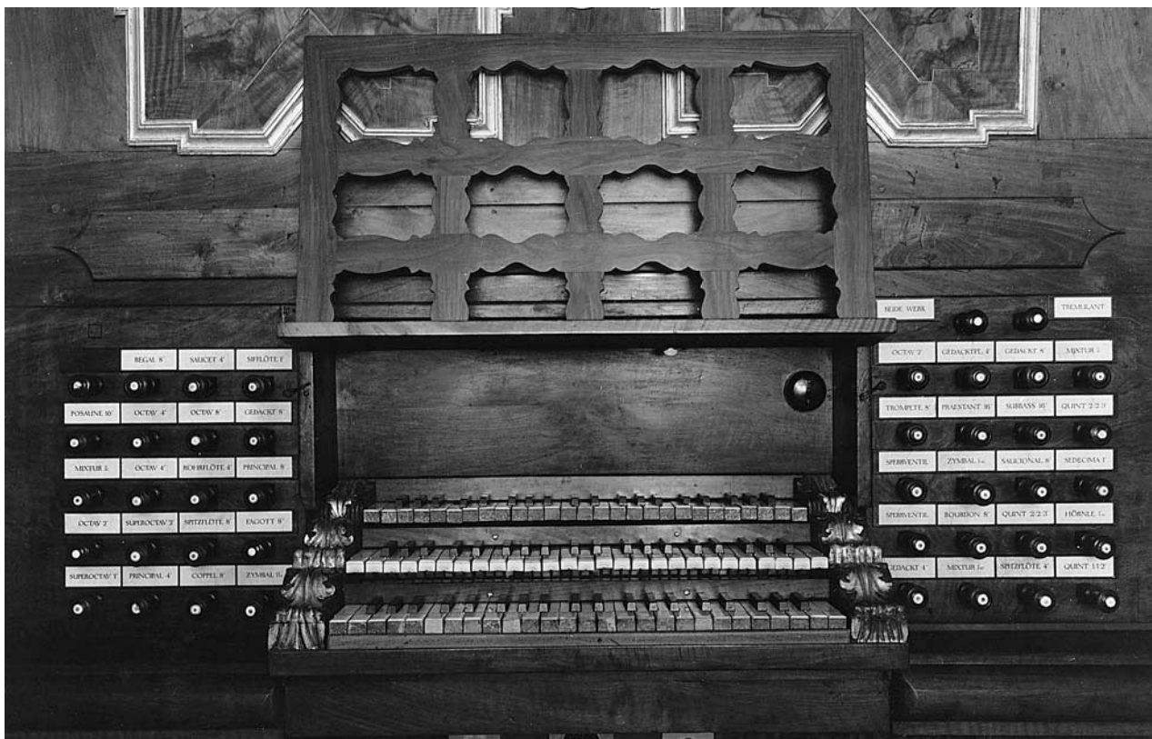
Abb. 70–72 Rheinau. Ehem. Klosterkirche. Hauptorgel. Spieltisch. Links: Der 1941 entfernte Spieltischkasten in geöffnetem Zustand. Historische Aufnahme vor 1941. Oben: Situation nach der Restaurierung 1941; die Staffeleibretter sind noch wie bei Haas auf der Gehäusefront angenagelt. Unten: Situation nach der Restaurierung 1988–1990; die Staffeleibretter sind wie vor Haas etwa um Brettstärke eingesenkt. Aufnahme von 1998.
