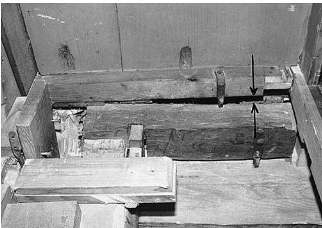
Abb. 78–79 Rheinau. Ehem. Klosterkirche. Hauptorgel. Rückpositiv. Links: Der Grundrahmen des Gehäuses wurde durch Einschnitte geschwächt und kippte nach vorne. Rechts: Im prospektseitigen Stück des Grundrahmens sind noch die Ausschnitte für die originalen Windladenlager zu sehen.
