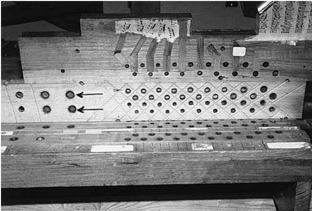
Abb. 42–43 Rheinau. Ehem. Klosterkirche. Hauptorgel. Links: Rückpositivwindlade mit aufgekippten Pfeifenstöcken. Oben orig. Prospektstock (Nussbaum) mit eingestimmten, sauber verspundeten Verführungen. Darunter neuer Stock (Eiche) von Haas mit Zusatzbohrungen im Fundament für Zusatzventile. Rechts: Zwei der von Haas eingebauten Zusatzventile im Rückpositiv. In diesem Bereich ist der Steg des Windkastens nachgeschnitten. Die Zusatzventile tragen, im Gegensatz zu den funktionellen Ventilen, auf der Stirnseite keine Tonbezeichnungen.
