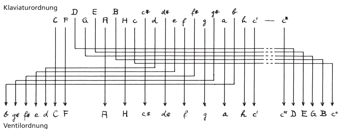
Abb. 135–136 Rheinau. Ehem. Klosterkirche. Chororgel. Oben: Stechermechanik mit Manualwellenbrett nach der Restaurierung, darunter die Abgänge der Pedaltraktur. Unten: Schema des original erhaltenen Manualwellenbrettes (nicht massstäblich). Die Klaviaturordnung entspricht der üblichen «kurzen Oktave» im Bass, die unkonventionelle Ventilordnung dagegen ist durch die besondere Gehäuseform bedingt. Nach dem Inventarbericht des Verfassers von 1962.
