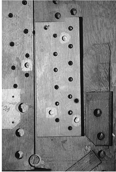
Abb. 123–124 Rheinau. Ehem. Klosterkirche. Chororgel. Pfeifenstock für Coppel 8', Diskant, mit dem Überstock für die neuen Metallpfeifen c 2 -c 3 von 1944. Nach der Ablösung des Überstockes wurden die Originalbohrungen für die Holzpfeifen c 2 -c 3 wieder sichtbar. (Abb. rechts).
