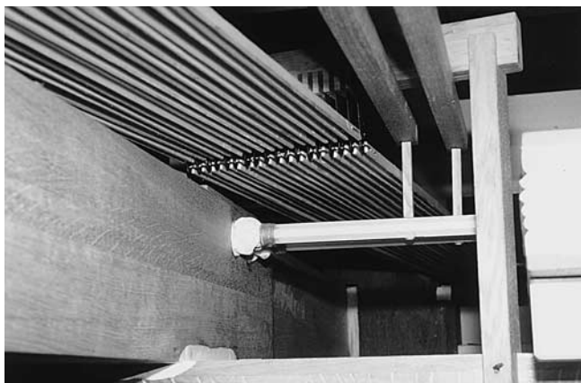
Abb. 138 Rheinau. Ehem. Klosterkirche. Chororgel. Umgelenkte Pedaltraktur unter dem Chorgestühl, rechts davon die beiden Pedalregisterzüge, verbunden mit zwei Sperrventilen im Windkanal.
