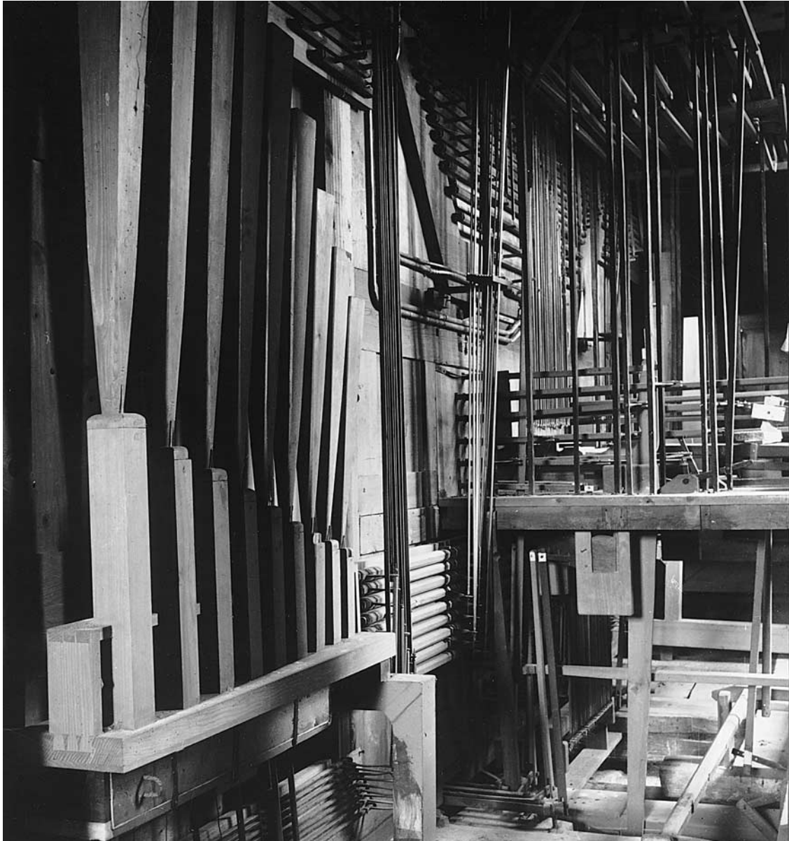
Abb. 47 Rheinau. Ehem. Klosterkirche. Hauptorgel. Seitlicher Blick in den Unterbau vor den Arbeiten 1941. Links unten die originale Separatlade für die Pedal-Posaune 8' Fuss von Leu samt Mechanik (D-Seite). Auf dem verbreiterten Pfeifenstock steht die hölzerne Pedaltrompete von Haas. Historische Aufnahme um 1940.
