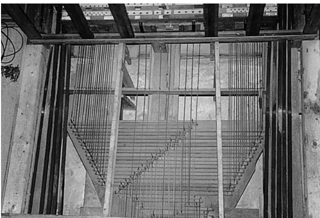
Abb. 58 Rheinau. Ehem. Klosterkirche. Hauptorgel. Wellenbrett des Rückpositivs, wohl seit dem Umbau von 1756 liegend unter dem Fussboden platziert; links und rechts davon die schweren eisernen Zugstangen der Registerzüge.
