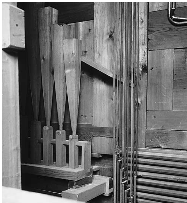
Abb. 48 Rheinau. Ehem. Klosterkirche. Hauptorgel. Blick von hinten in den Unterbau, vor den Arbeiten 1941. Erkennbar die originale Windeinspeisung für die Separatlade. Haas verwendete für die durchschlagende Pedalalange abgestimmte hölzerne Stiefel. Historische Aufnahme um 1940.
