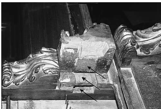
Abb. 55 Rheinau Ehem. Klosterkirche. Hauptorgel. Linker Klaviaturbacken des I. Manuals, von innen betrachtet; der obere Teil ist hochgekippt. Der Durchgang für die originale Schiebekoppelbetätigung zeigt noch Reste von textilem Belag.
