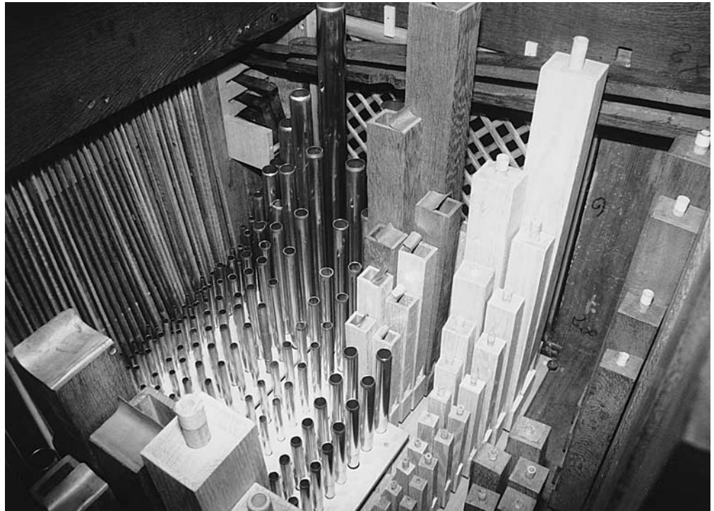
Abb. 119 Rheinau. Ehem. Klosterkirche. Chororgel. Blick in das fertig restaurierte bzw. rekonstruierte Pfeifenwerk, links die Stechermechanik des Manuals.
