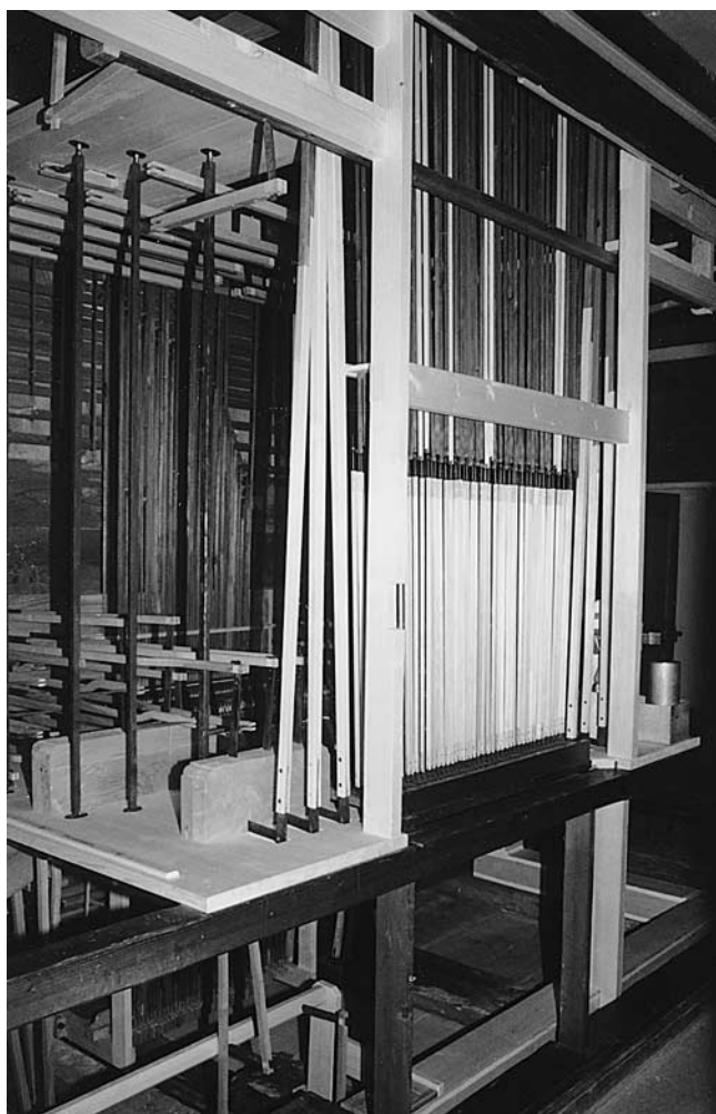
Abb. 60 Rheinau. Ehem. Klosterkirche. Hauptorgel. Die Wippen zur Betätigung der Oberwerktraktur ruhten vor der Restaurierung direkt auf den hinteren Enden der Tasten des III. Manuals, mit einer Belederung zur Lärmdämpfung. Da und dort sind noch Reste einer ursprünglichen Pergamentumfassung der Wippenenden zu sehen.
