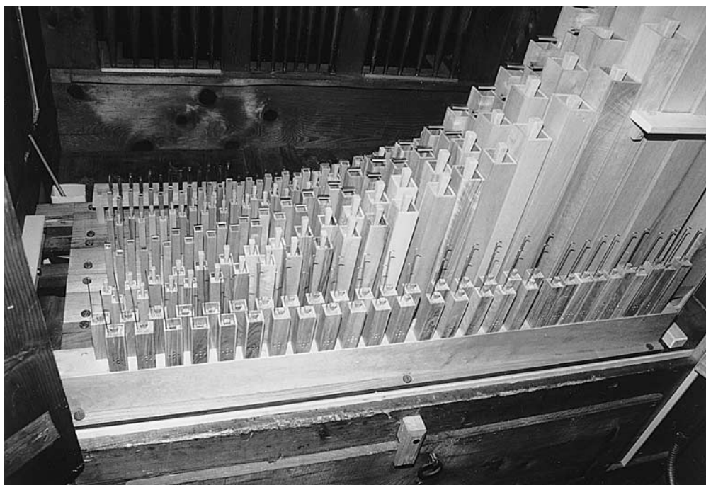
Abb. 32 Rheinau. Ehem. Klosterkirche. Hauptorgel. Blick ins restaurierte Pfeifenwerk des Pedals. Rechts die neuen Subbasspfeifen mit den Nussbaumeinsätzen, links eine grosse Innenpfeife des Prospektregisters.
