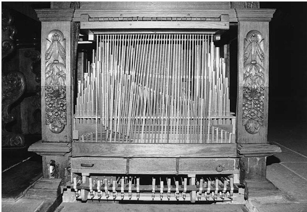
Abb. 134 Rheinau. Ehem. Klosterkirche. Chororgel. Die Spieltischfront ohne die Kniefüllung, vor der Restaurierung. Stechermechanik und Manualwellenbrett. Am Gehäuse sind die 1944–1945 ergänzten Schnitzereien (anstelle der Registerstaffeleien) gut zu erkennen.
