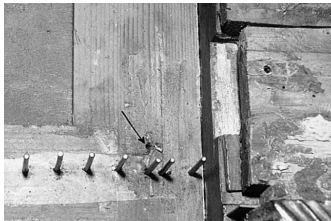
Abb. 53–54 Rheinau. Ehem. Klosterkirche. Hauptorgel. Die Klaviaturrahmen des I. Manuals nach Ausbau der Tasten, Bass- und Diskantseite. Der Rahmen liegt lose zwischen den seitlichen Klaviaturbacken und zeigt deutliche Befestigungsspuren der originalen Schiebekoppelvorrichtung.
