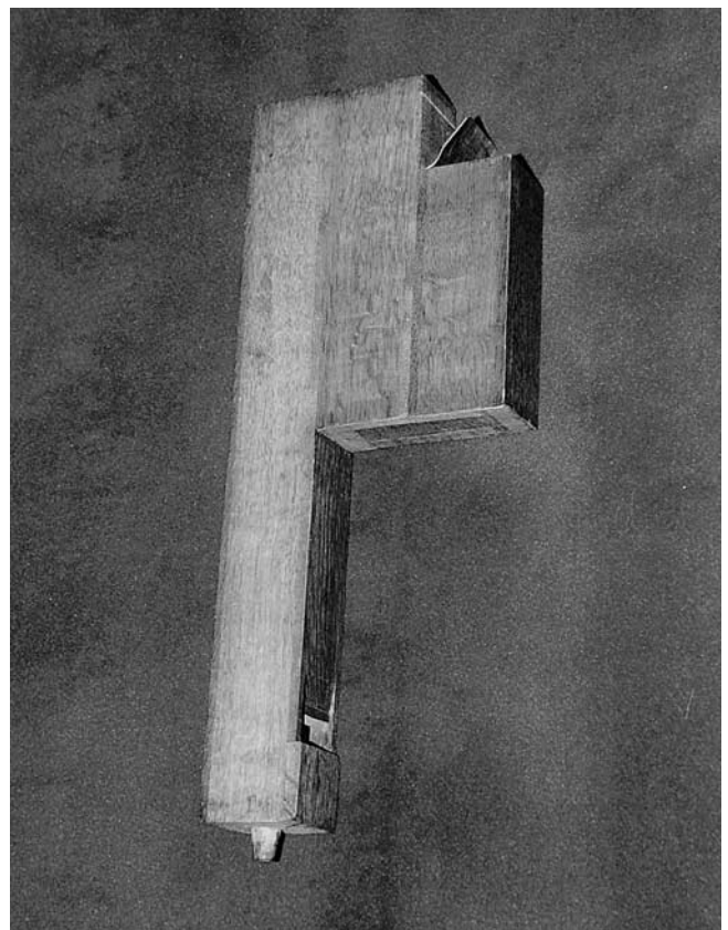
Abb. 120 Rheinau. Ehem. Klosterkirche. Chororgel. Mehrfach gekröpfte Holzpfeife des Registers Principal 8', original erhaltener Ton cis 0 .
