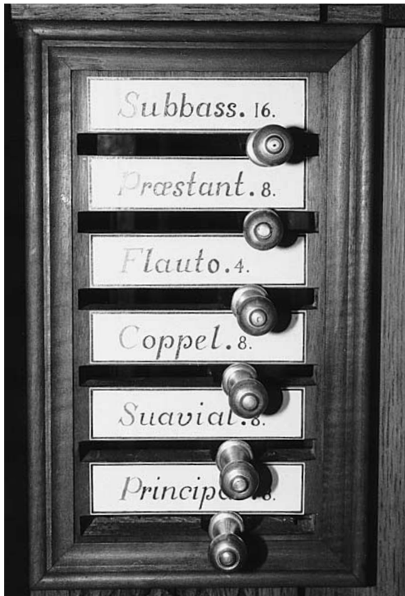
Abb. 141–144 Rheinau. Ehem. Klosterkirche. Chororgel. Oben: Nach den Originalen neu hergestellte Registerstaffeleien am fertig restaurierten Instrument, jetzt sauber konzipiert für zwölf Register. Unten: Restaurierte Registermechanik von innen betrachtet. Links die Diskantseite mit sechs abgekröpften Registerzügen. Rechts die Basseite mit vier abgekröpften Manualregisterzügen und den zwei nicht abgekröpften Pedalregisterzügen.
