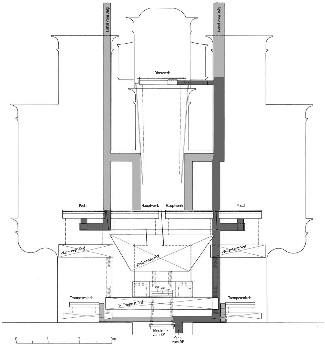
Abb. 77 Rheinau. Ehem. Klosterkirche. Hauptorgel. Rekonstruierte Kanalanlage von Leu mit zwei ungleich dimensionierten vertikalen Hauptkanälen vom Dachboden zur Orgel. Dunkelgrau gerastert die noch in situ erhaltenen Kanäle, hellgrau die Ergänzungen der jüngsten Restaurierung. Aufriss der Werkanordnung nach der Restaurierung 1988–1990, mit Windladen- und Wellenbrettpositionen sowie Trakturverläufen. Schnitt durch die Anlage vgl. Abb. 106. Orgelbau Th. Kuhn AG, Männedorf, 1992.
