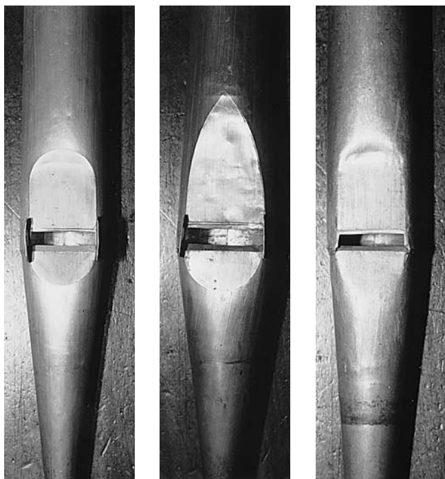
Abb. 27–29 Rheinau. Ehem. Klosterkirche. Hauptorgel. Die drei verschiedenen, von Leu gefertigten Labientypen. Links: Rundlabien oben und unten. Mitte: Spitzlabium oben und Rundlabium unten. Rechts: auslaufende Labien.
