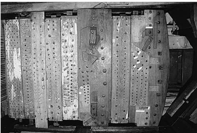
Abb. 125–126 Rheinau. Ehem. Klosterkirche. Chororgel. Links: Gesamtansicht der Manuallade. Zustand nach Entfernung der neueren Überstöcke und Deckfurniere, jedoch vor der weiteren Restaurierung. Rechts: Windladenoberseite, abgebaut bis auf den belederten Schleifengrund. Zweite Schleifenbahn von rechts: das Diskantregister Suavial 8' beginnt erst bei c 1 .
