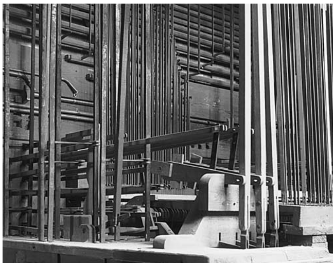
Abb. 64 Rheinau. Ehem. Klosterkirche. Hauptorgel. Aufnahme der Mechanik vor 1941 mit den schweren Vierkanteisen der Registermechanik, dem Hauptwerkwellenbrett und rechts dem Abgang der Oberwerkstraktur. An der Gehäuserückwand sind links die drei Löcher für die zusätzlichen Pedalregister von 1756 zu sehen, rechts die drei Löcher für die Oberwerksregister. Historische Aufnahme um 1940.
