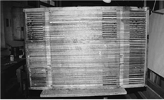
Abb. 127 Rheinau. Ehem. Klosterkirche. Chororgel. Freigelegte Unterseite der Manuallade, rechts aussen die Klaviaturseite mit den 45 Tonventilschlitzern, links aussen die 18 Schlitz für die Koppelventile des Pedals. Die 18 zusätzlichen Ventilschlitz hinter den Manualventilen sind funktionslos.
