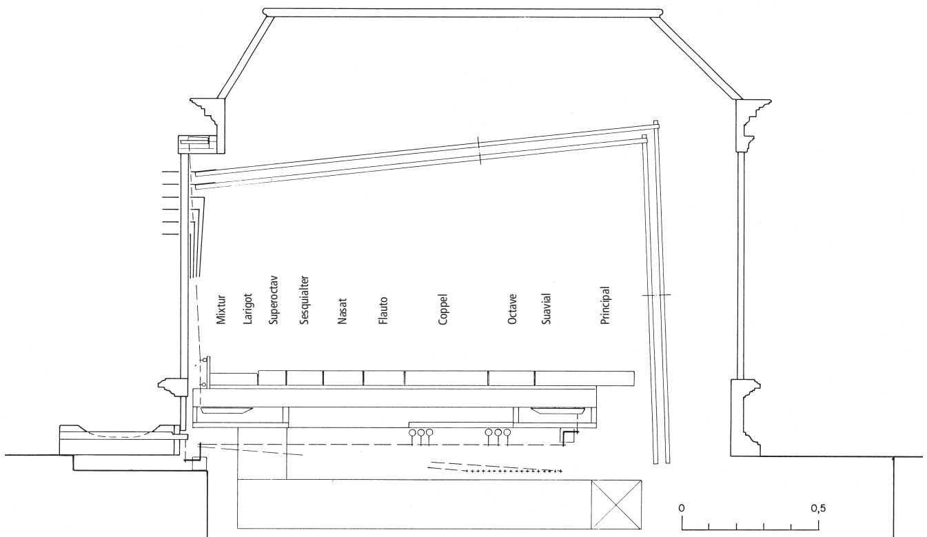
Abb. 152–153 Rheinau. Ehem. Klosterkirche. Oben: Querschnitt durch die Gesamtanlage, Gebläse unter dem dreistufigen Chorgestühl, Pedalwerk hinter dessen Rückwand. Unten: Längsschnitt mit Windladenposition, Stellung der Register auf der Lade, Trakturverlauf und Windkanal. Pläne Orgelbau Th. Kuhn AG, Männedorf, 1992.
