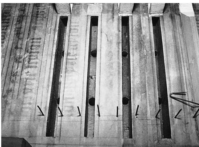
Abb. 40–41 Rheinau. Ehem. Klosterkirche. Hauptorgel. Oben: Ausgebaute Windlade des Rückpositivs vor der Restaurierung; Reparaturinschrift von Haas 1840/1841. Unten: Rückpositivwindlade nach Ausbau der Ventile, Blick in die Tonkanzellen. In den zwei Kanzellen links ist die neue eichene Fundamentplatte von Haas zu sehen, in den zwei Kanzellen rechts sind noch nussbaumene Verspundungen von Leu erhalten geblieben. Originale Pergamentbespannung der Ladenunterseite mit alten Choralhandschriften.
