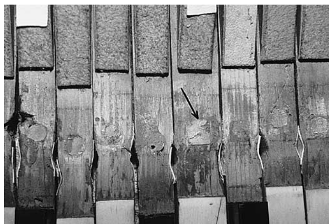
Abb. 56 Rheinau. Ehem. Klosterkirche. Hauptorgel. Ausgebaute Tasten des I. Manuals. Gut erkennbar sind Reste der originalen quadratischen Kopplungsstecherklötzchen sowie runde Dübelausflicke.
