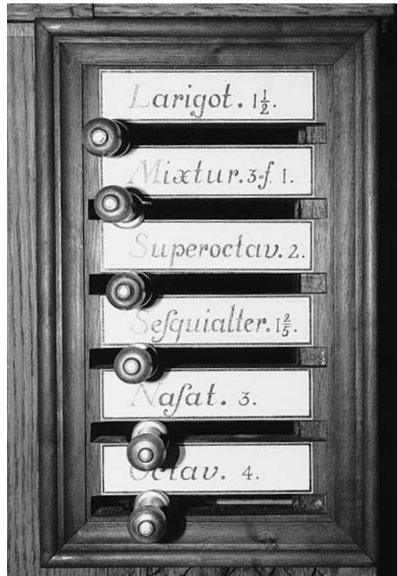
Abb. 141–144 Rheinau. Ehem. Klosterkirche. Chororgel. Oben: Nach den Originalen neu hergestellte Registerstaffeleien am fertig restaurierten Instrument, jetzt sauber konzipiert für zwölf Register. Unten: Restaurierte Registermechanik von innen betrachtet. Links die Diskantseite mit sechs abgekröpften Registerzügen. Rechts die Basseite mit vier abgekröpften Manualregisterzügen und den zwei nicht abgekröpften Pedalregisterzügen.
