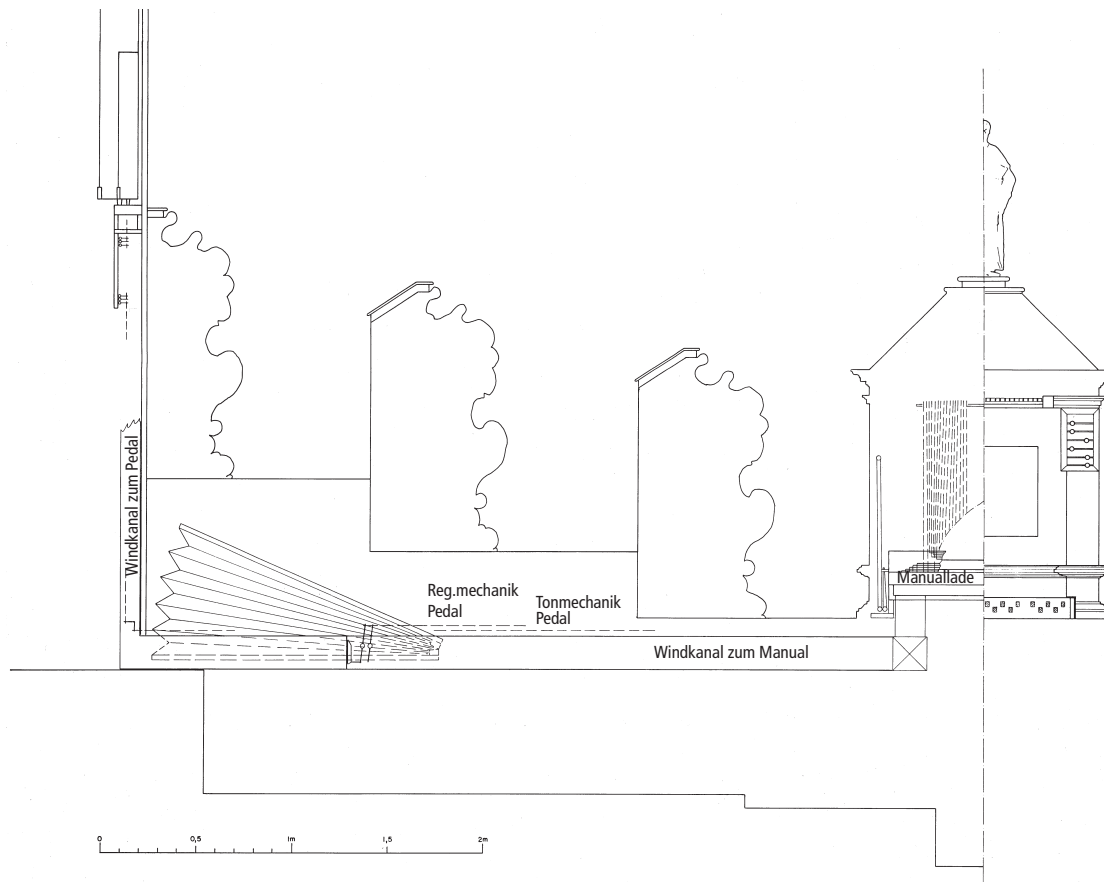
Abb. 152–153 Rheinau. Ehem. Klosterkirche. Oben: Querschnitt durch die Gesamtanlage, Gebläse unter dem dreistufigen Chorgestühl, Pedalwerk hinter dessen Rückwand. Unten: Längsschnitt mit Windladenposition, Stellung der Register auf der Lade, Trakturverlauf und Windkanal. Pläne Orgelbau Th. Kuhn AG, Männedorf, 1992.
