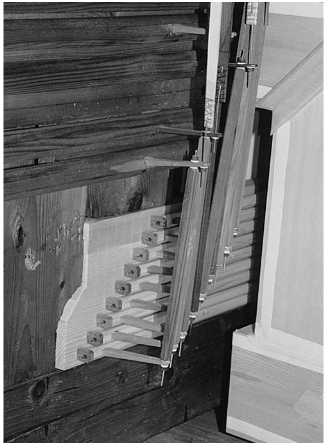
Abb. 50 Rheinau. Ehem. Klosterkirche. Hauptorgel. Rekonstruierte Abzweigung der Pedalmachanie. Nach oben verläuft die normale Abstraktenmechanik zur Pedallade, nach unten zweigt die Stechermechanik zur Separatlade der Pedalposaune ab.
