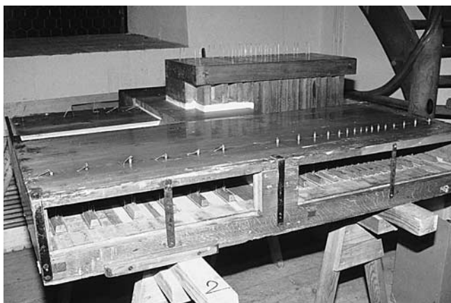
Abb. 38–39 Rheinau. Ehem. Klosterkirche. Hauptorgel. Links: Erweiterung der Windeinspeisung durch Haas; ausgebaute Hauptwerkslade umgekehrt auf Böcken lagernd. Im Bassteil links ein zweiter Ventilkasten, im Diskantenteil rechts eine Zusatzlade mit Holzkondukten zur Hauptlade. Rechts: Die Zusatzlade ist abgehoben und aufgestellt. Die Holzkondukten leiten den Zusatzwind aus der Zusatzlade in die Kanzellen der originalen Hauptlade.
