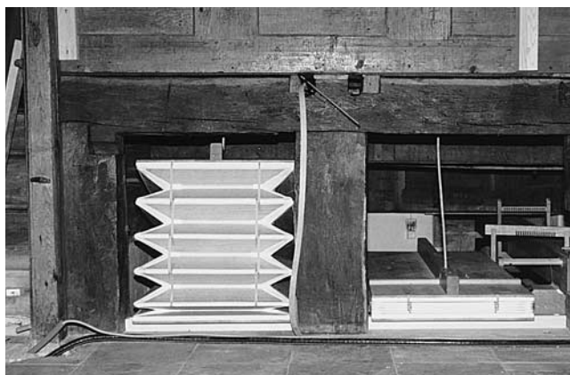
Abb. 146–147 Rheinau. Ehem. Klosterkirche. Chororgel. Oben: Anhand der Spuren rekonstruierte doppelte Keilbalganlage unter dem Chorgestühl, mit Seilzug über Rollen. Unten: Blick von aussen auf die rekonstruierte Balganlage, ohne Rückwand. In der Mitte oben die zwei originalen Löcher für die ledernen Zugriemen, rechts aussen die Aufhängeraster für die (noch nicht montierte) Pedalmechanik.
