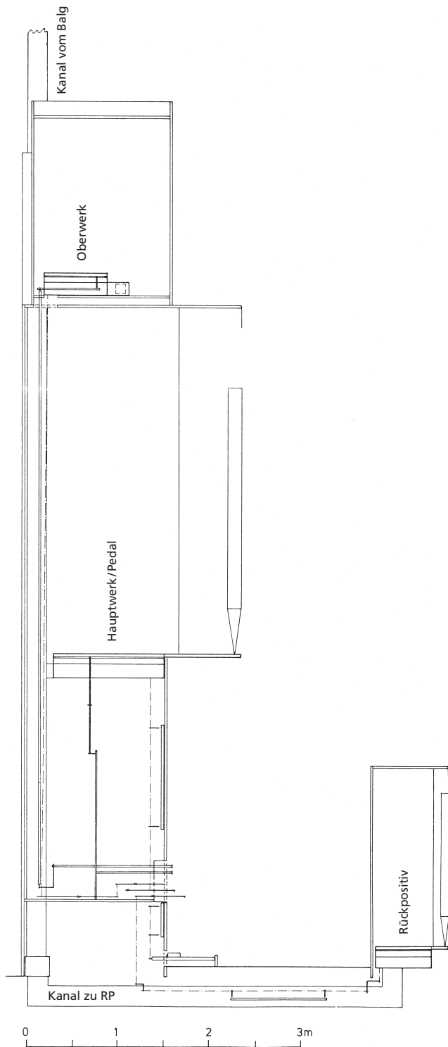
Abb. 106 Rheinau. Ehem. Klosterkirche. Hauptorgel. Schnitt durch das restaurierte Instrument, mit Windladen- und Wellenbrettpositionen sowie Trakturverläufen. Plan Orgelbau Th. Kuhn AG, Männedorf, 1992. Vgl. Abb. 77 (Aufriss).
