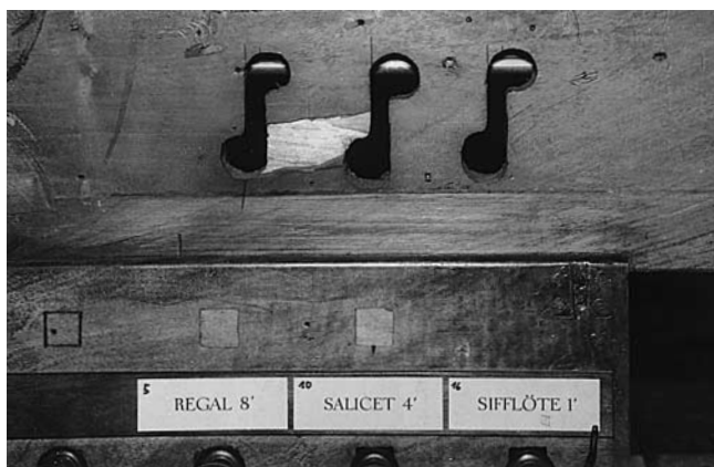
Abb. 62–63 Rheinau. Ehem. Klosterkirche. Hauptorgel. Links: Unter einer Deckleiste, deren Umrisse sichtbar sind, verbergen sich auf der linken Spieltischseite drei s-förmige Schlitzte zum Einhaken von drei Oberwerksregistern. Rechts: Auf der rechten Spieltischseite befinden sich ebenfalls drei Löcher zum Einhaken von drei Oberwerksregistern; zusammen also sechs. Rechts aussen übereinander gestellt drei viereckige Löcher für die drei zusätzlichen Pedalregister von 1756. Das oberste, durch die Zierleiste nicht verdeckte Loch ist sauber ausgeflickt.
