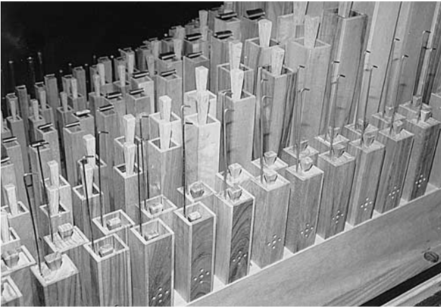
Abb. 34 Rheinau. Ehem. Klosterkirche. Hauptorgel. Das rekonstruierte Pfeifenwerk des Oberwerks, im Vordergrund das Geigenregal 8' mit hölzernen Resonatoren.
