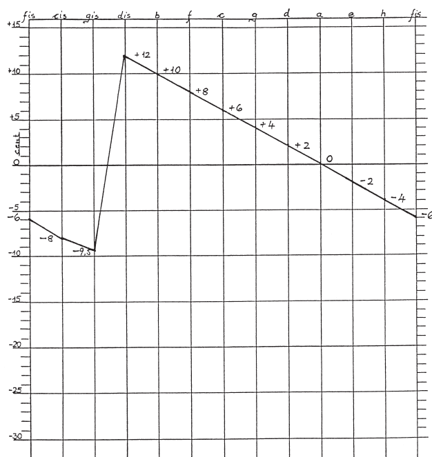
Abb. 105 Rheinau. Ehem. Klosterkirche. Hauptorgel. Das anhand der Versuche an den Prospektpfeifen erarbeitete Temperierungssystem, das für die Restaurierung schliesslich angewandt wurde. Grafik Orgelbau Th. Kuhn AG, Männedorf, 1992.
