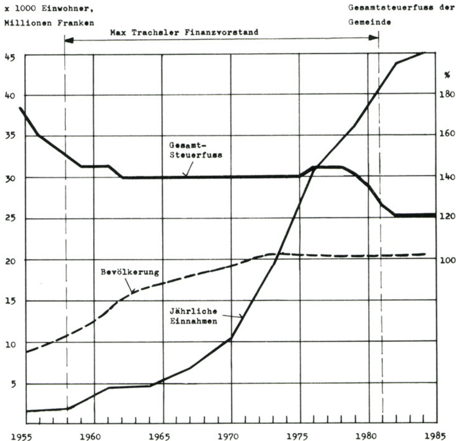
Gesamt-Einnahmen der politischen Gemeinde Dübendorf, Zahl der Einwohner und Gesamtsteuerfuss der Gemeinde in % von 1955 - 1985
