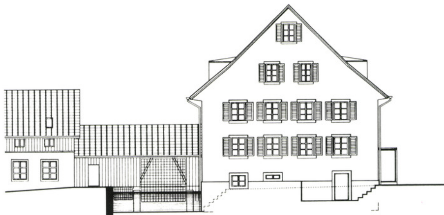
NORDWESTFASSADE
