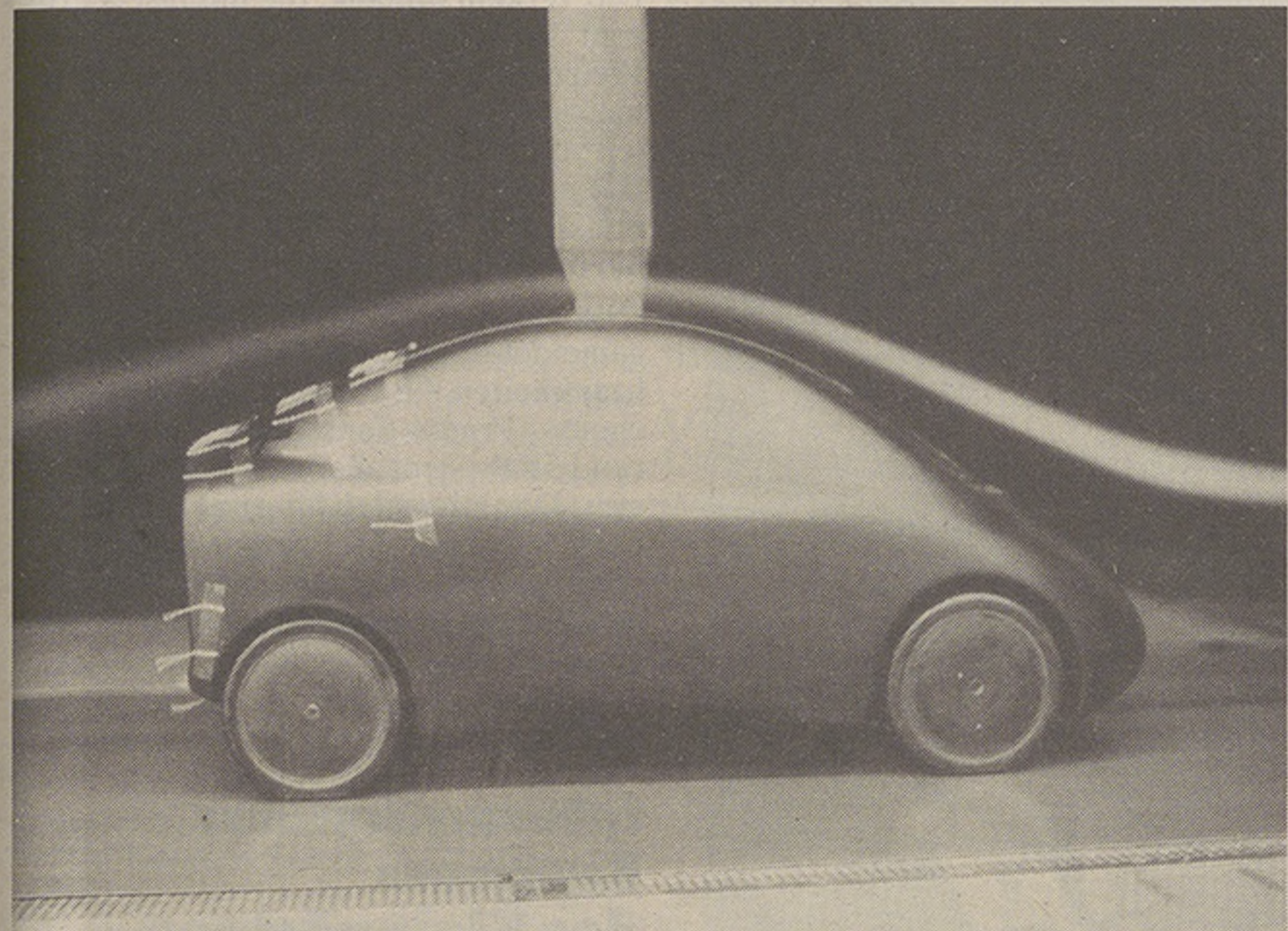
Im November 1992 soll der ESORO E301 der Öffentlichkeit vorgestellt werden. Das Bild zeigt den Prototypen im Windkanal.
