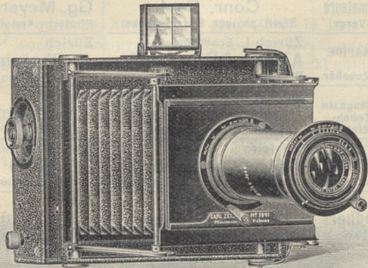
Minimum-Palmos 9 x 12 mit Tessar 1/6.3 f = 145 mm und Teleansatz I, fertig zur Teleaufnahme.
