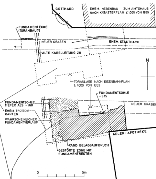
Altstadt. Untertor. Fundamente des ehem. Untertors. Übersichts-plan.
