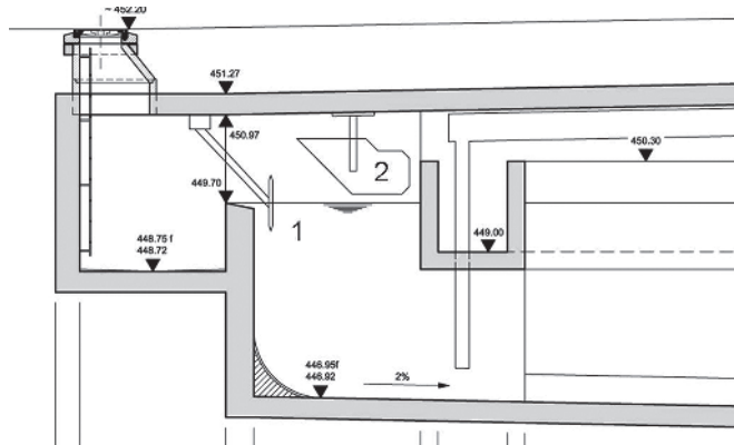
Teilschnitt durch das Regenbecken: 1 Tauchwand hält Schwimmteile zurück 2 Die Spülkippe zur Reinigung der Sohle
