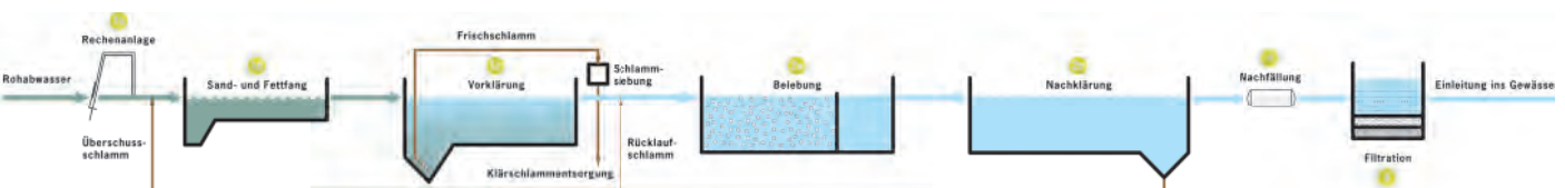
Die Abwasserreinigungsanlage im Hard reinigt in mehreren Stufen
