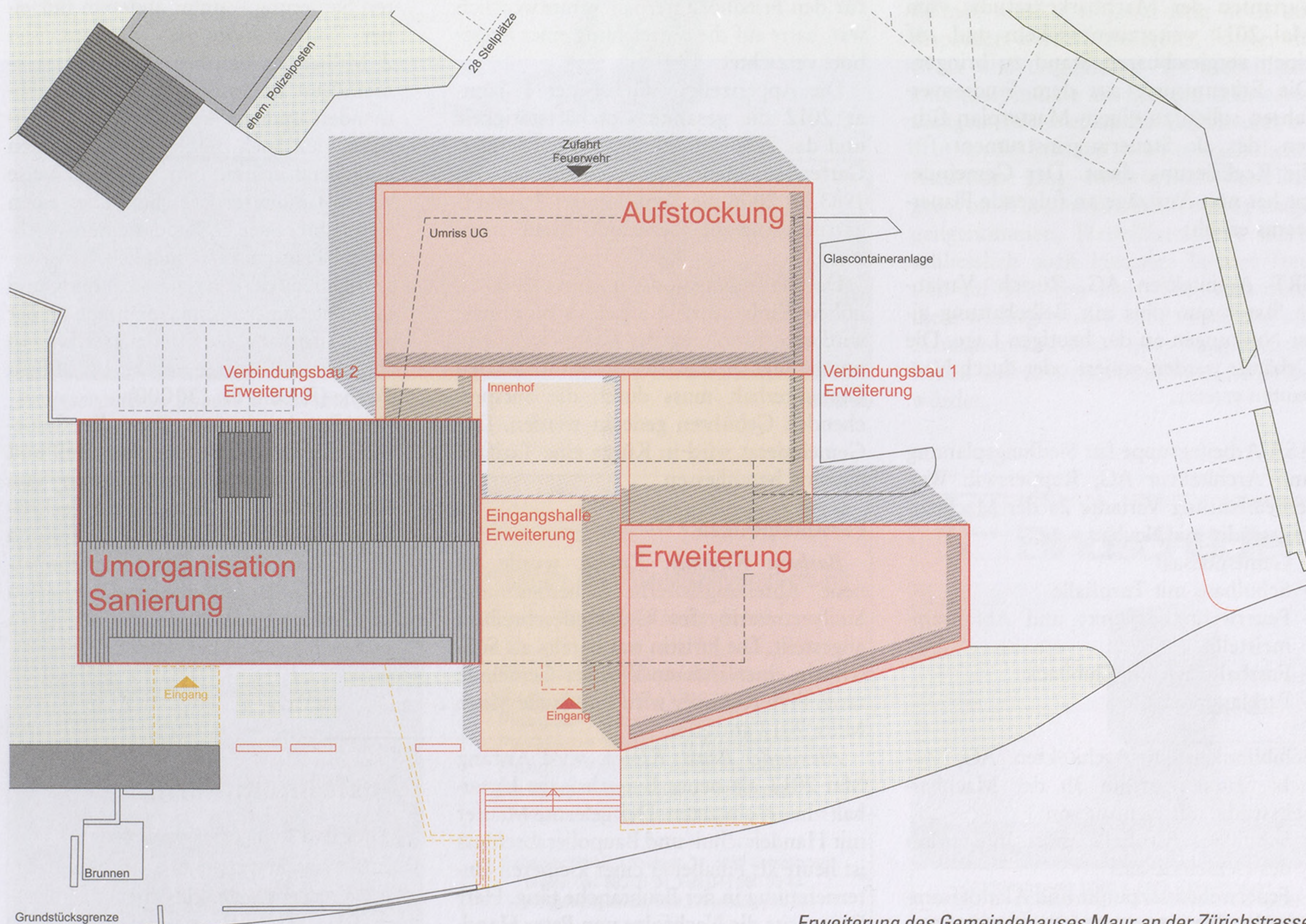
Erweiterung des Gemeindehauses Maur an der Zürichstrasse.
